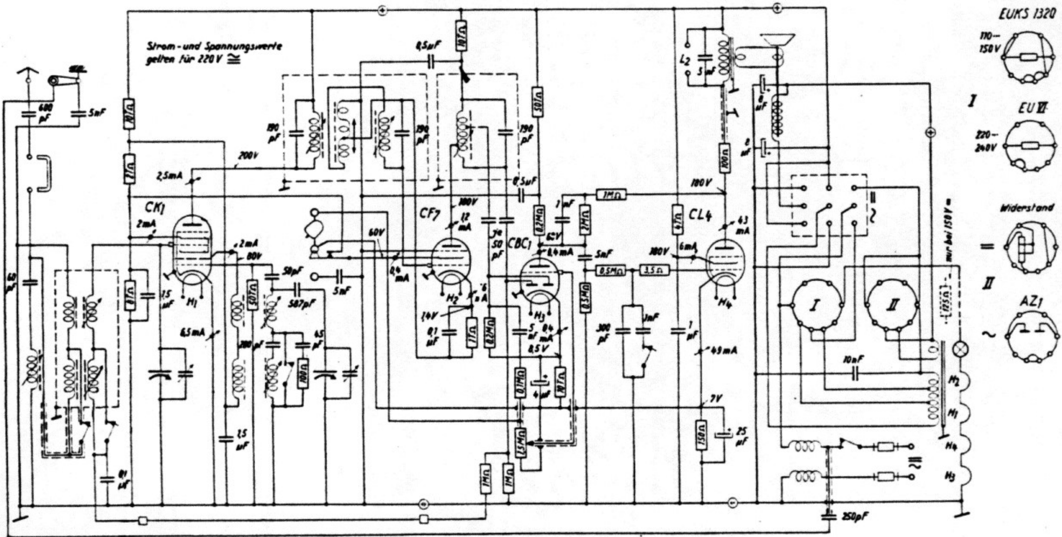
AEG, 57 GW, und Telefunken, 755 GW Markstein-Super, Allstrom, 1 Vorkreis, 3 Zwischenfrequenzkreise
