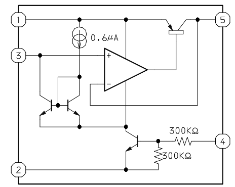
IC, TC7W74FU
