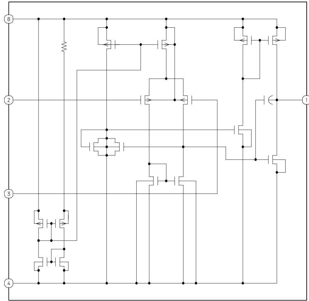
IC, NJU7014R-TE2
