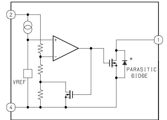
IC, S-8080ANNP
