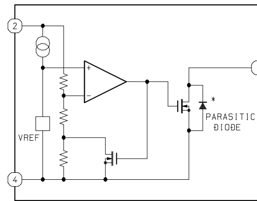
IC, S-80822ANNP
