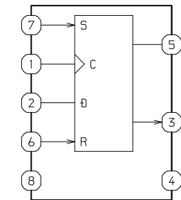
IC, TC7W74FU
