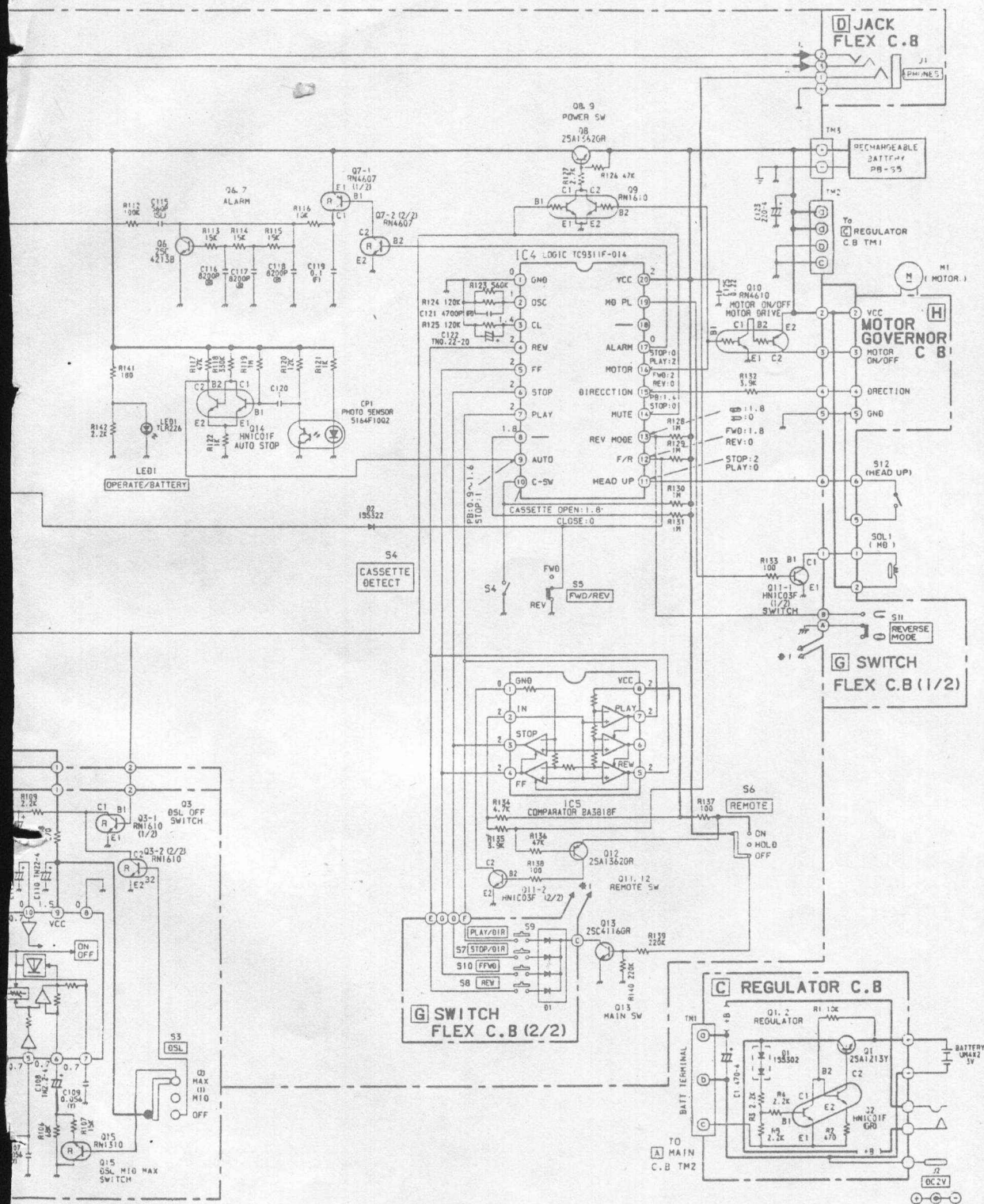
5 型随身听电路原理图
