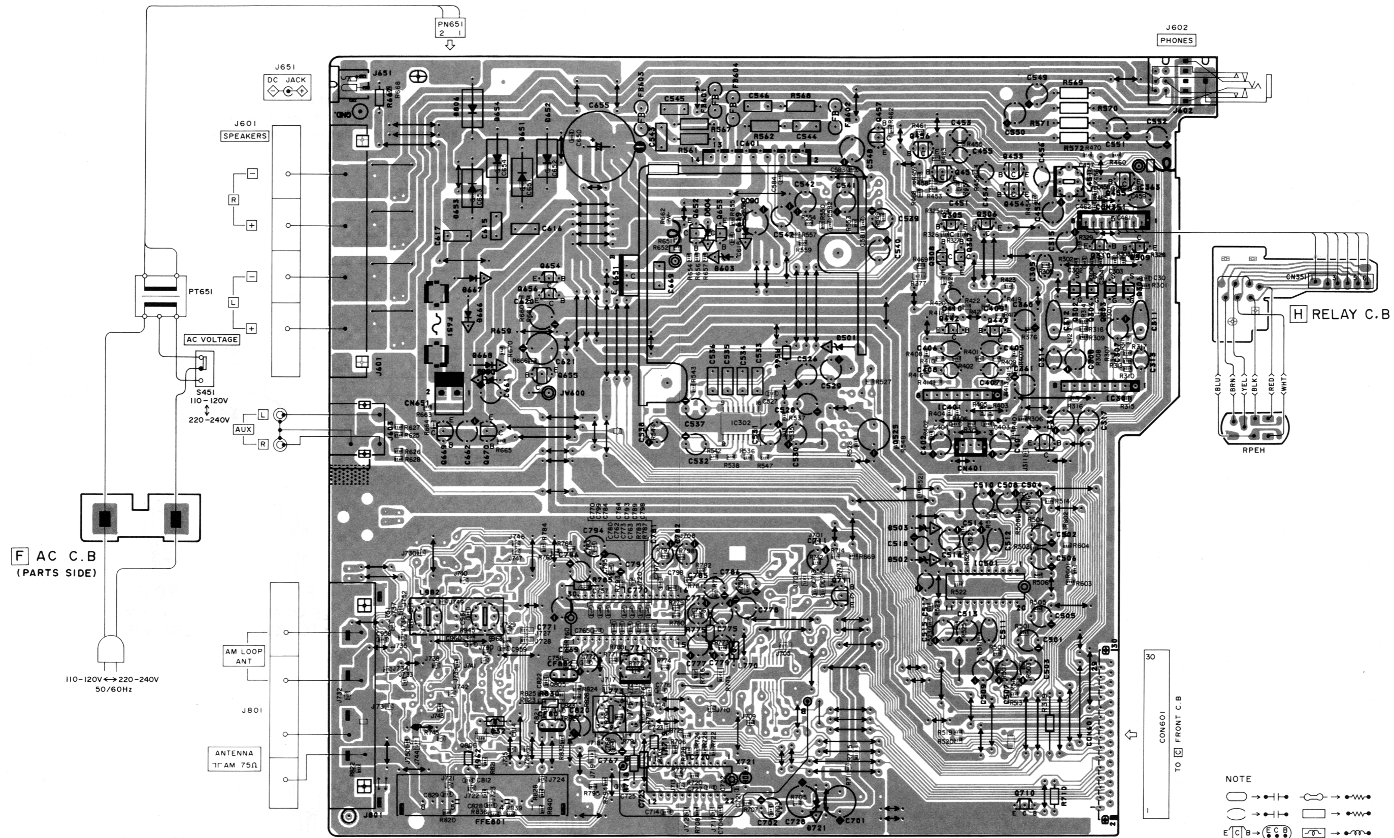
A MAIN C.B (PARTS SIDE)
