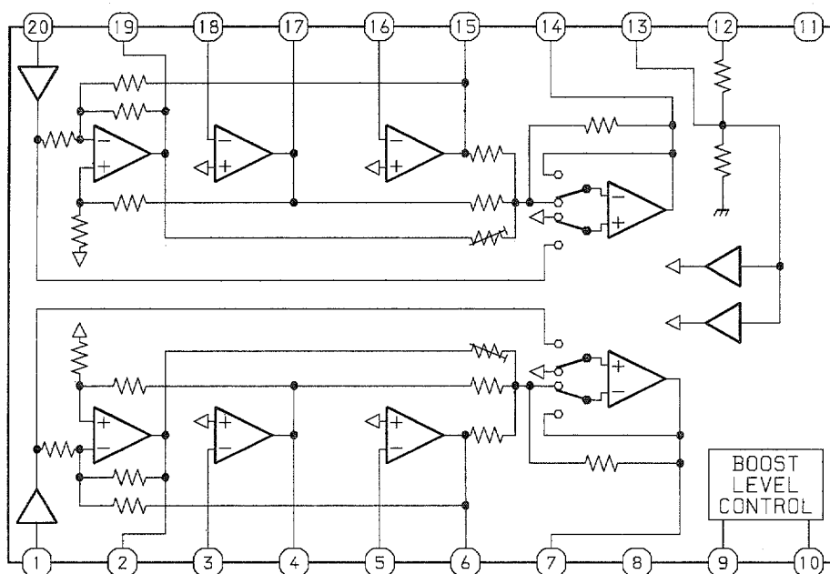
IC, NJM2152M
