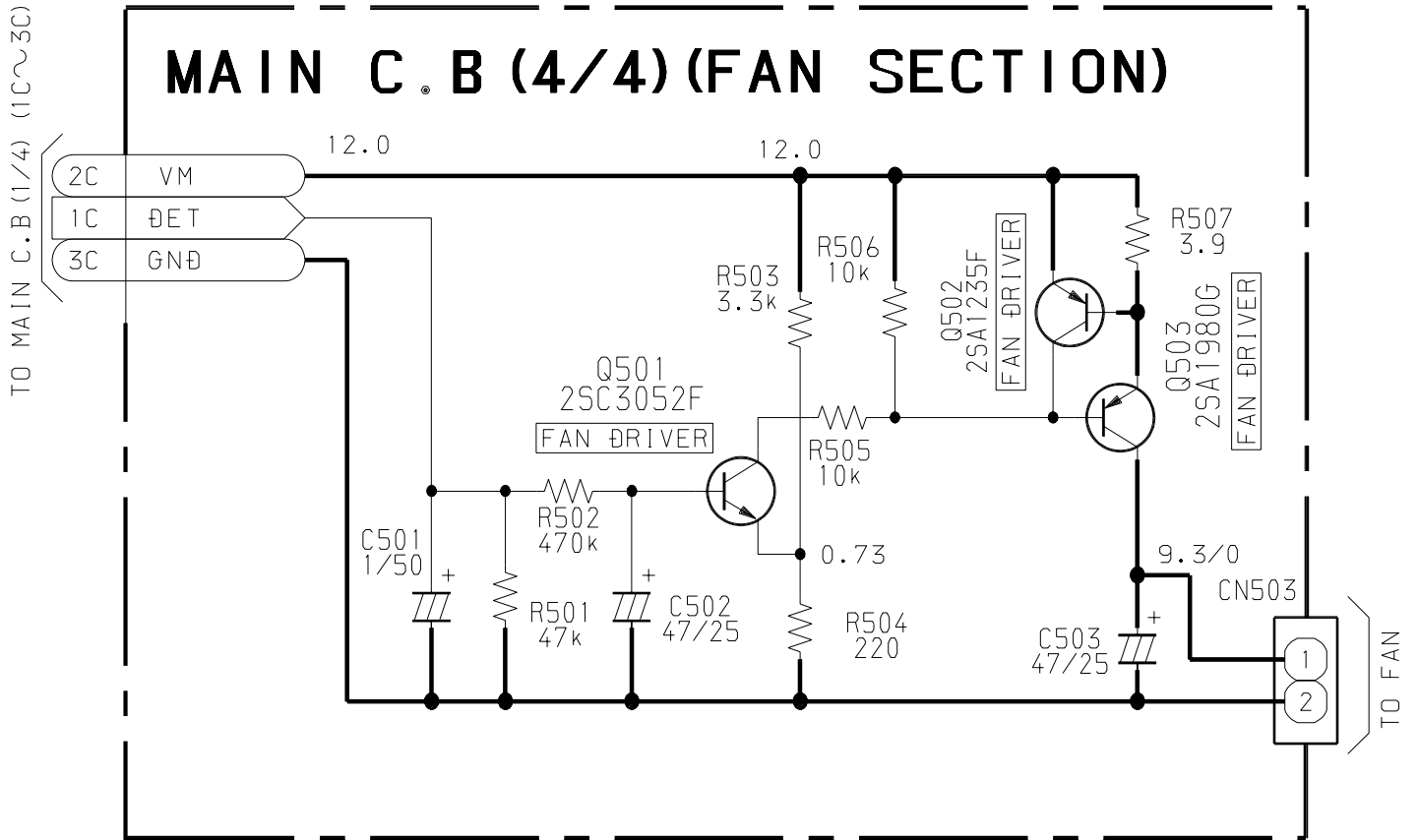
SCHEMATIC DIAGRAM – 4 (MAIN 4 / 4 : FAN SECTION)
