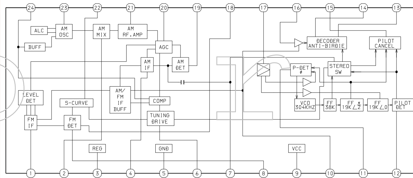
IC, LA1845N-A
