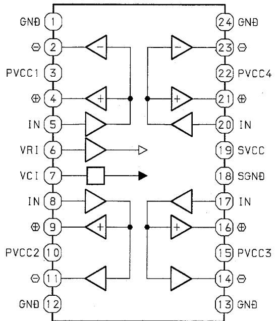
IC, TA2092N
