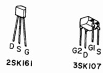
2SK161 3SK107
