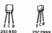
25C930 25C2999
