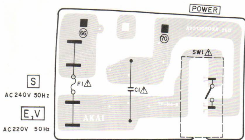
POWER PCB A2013D5072(AM-U41) A2013D5073(AM-U61)
