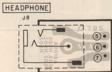
HEADPHONE PCB (U) A2018A503H (J) A2018A502H (C,A) A2018A504H (E,V,B,S) A2018A505H
