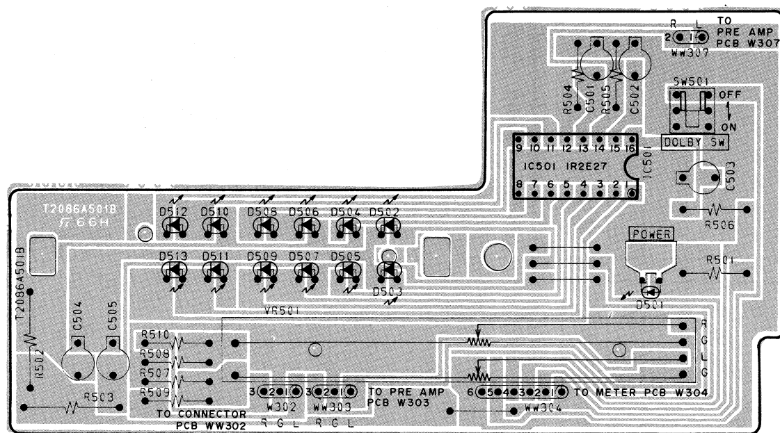
METER PCB T2086A501B
