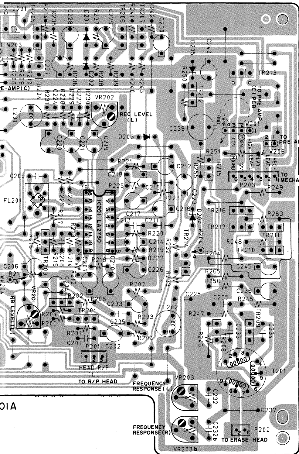
METER PCB
