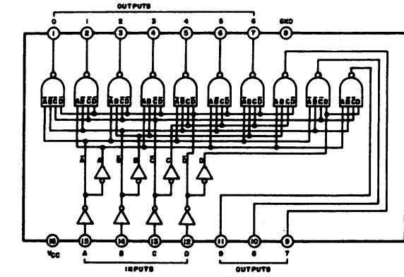
74LS42
