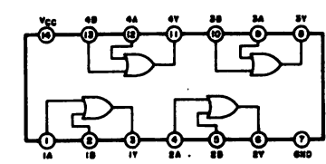
74HC32
