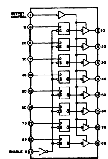
74LS373N
