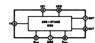
MN3009
