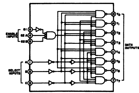
74HC138
