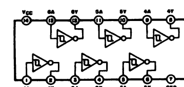
74LS14N
