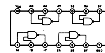
74HC38
