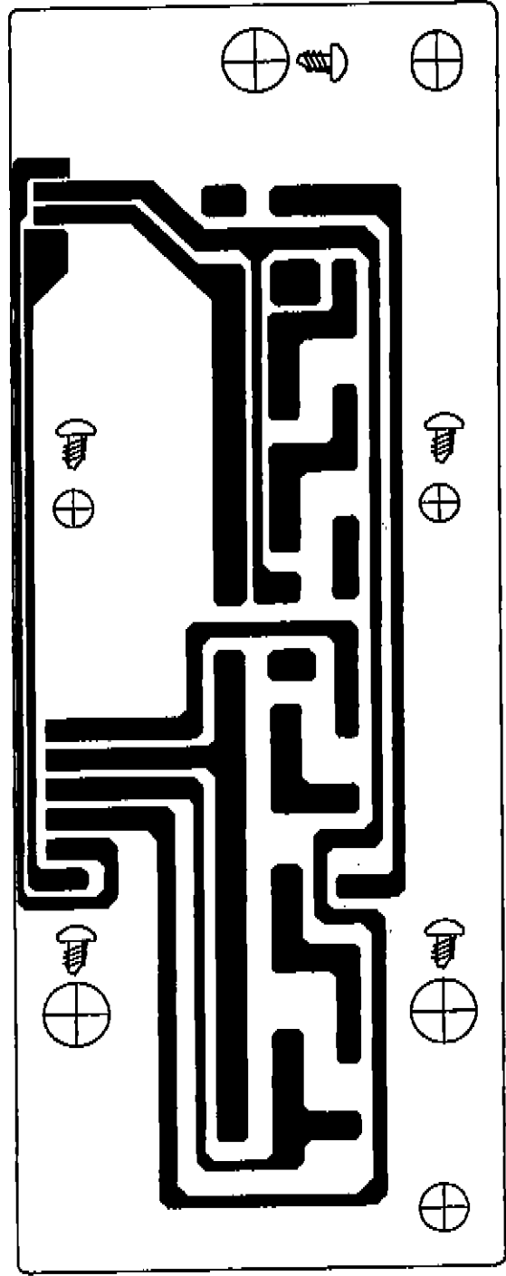
KEY-B PCB
