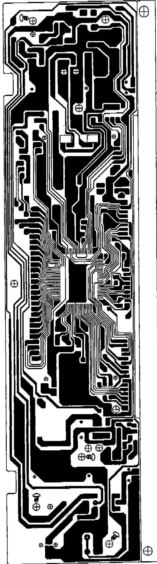
DISPLAY PCB
