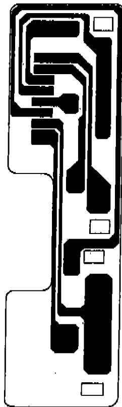
AUX PCB
