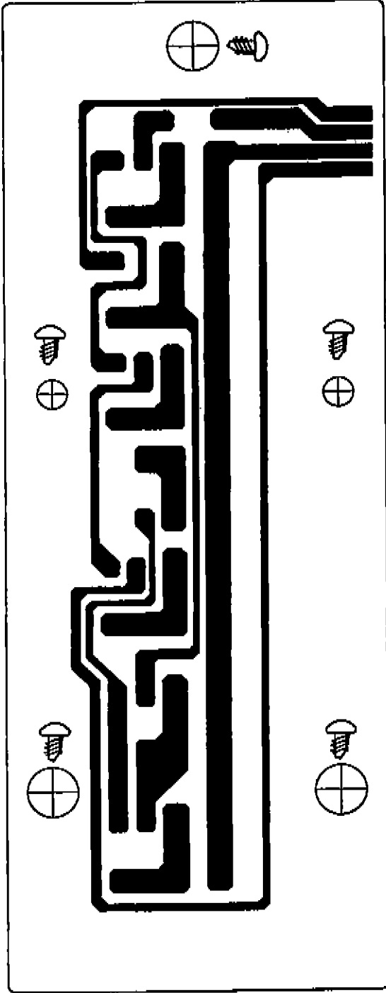
KEY-A PCB
