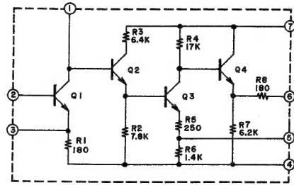
TA7139
