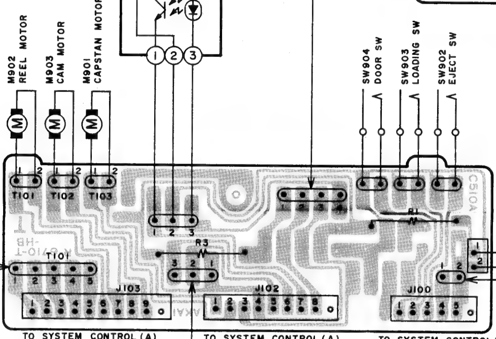
コントロール(B)A基板 CNTROL(B) A PCB CMR30C510A
