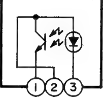
ガイド検出基板 GUIDE DETECTOR PCB CMR01B0050
