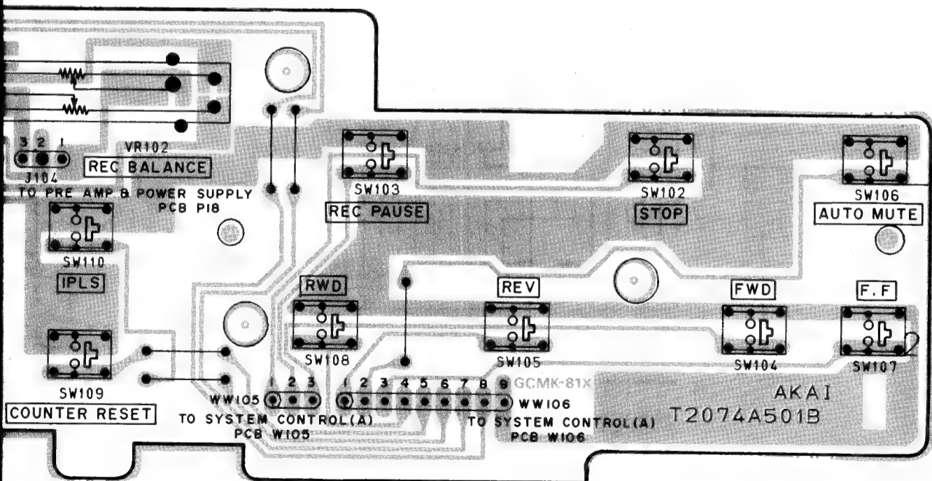
METER PCB T2074A501B メーター基板
