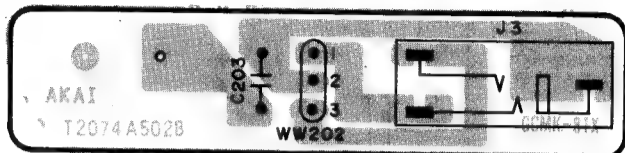
ヘッドホン基板 HEAD PHONE PCB T2074A502B
