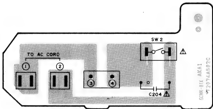
POWER SW PCB T2074A502C 電源スイッチ基板
