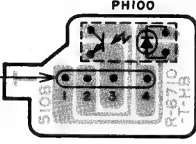
コントロール(B)B基板 CNTROL(B) B PCB CMR30C510B
