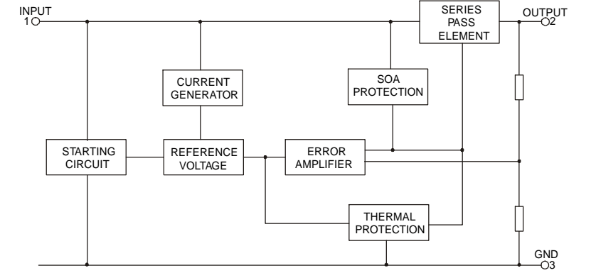
IC309 L7806CV
