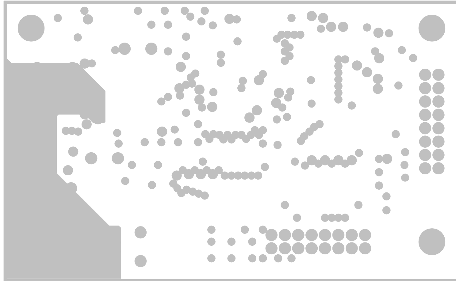
313123/2 II' INTERNAL LAYER VCC
