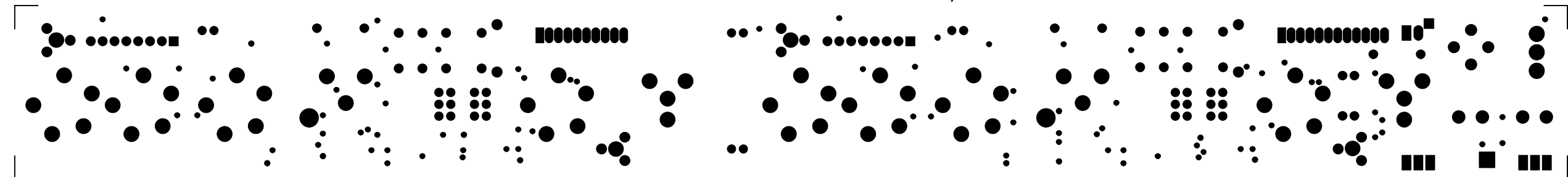
PCB : CLE20-PU Bottom Solder Mask
