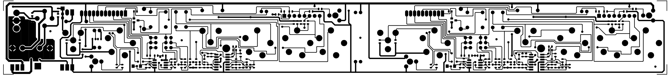
PCB : CLE20-PU Top Layer
