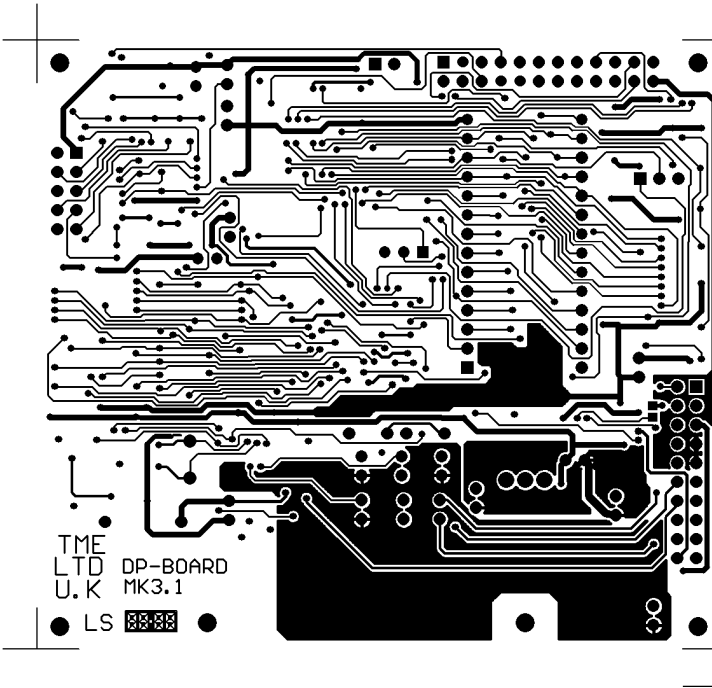
BOTTOM LAYER
