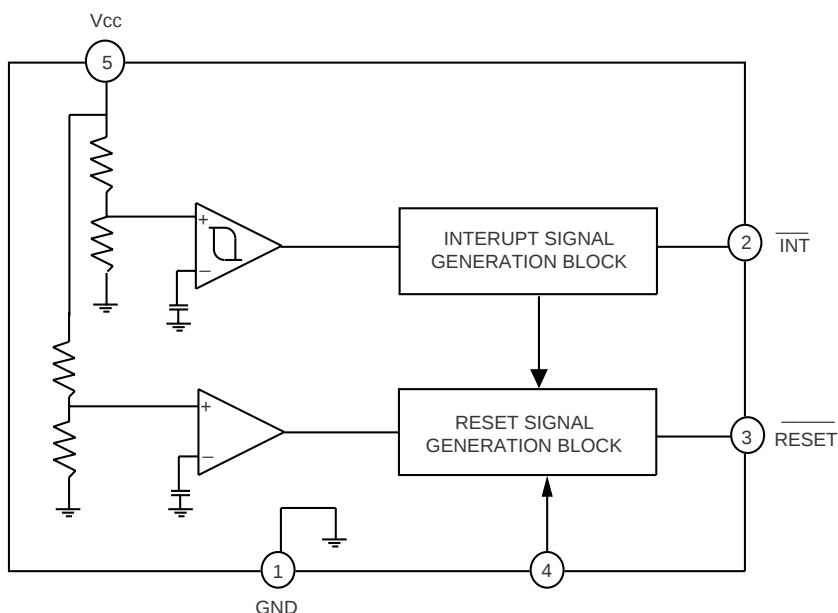
IC 604 (M62007FP)
