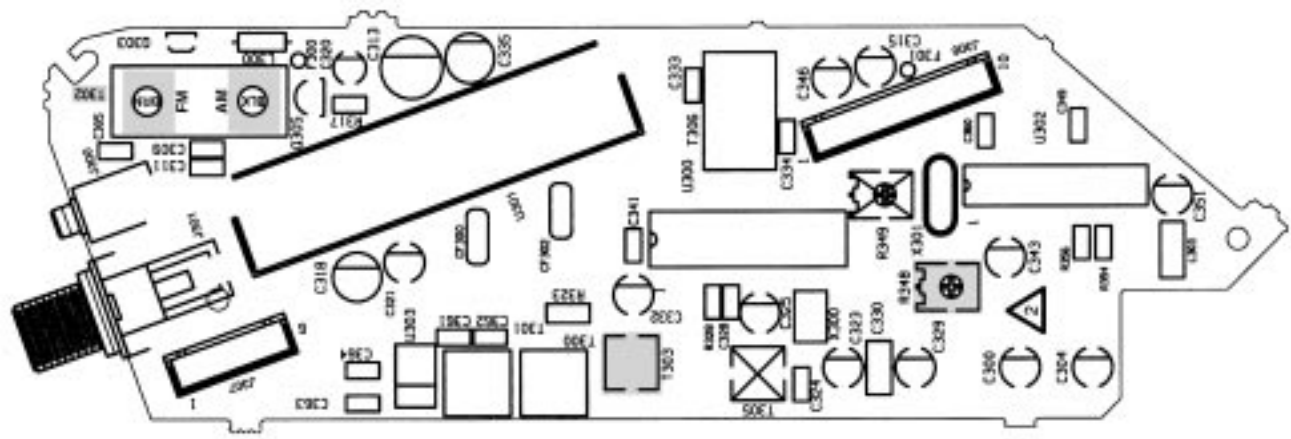
PCB 250736
