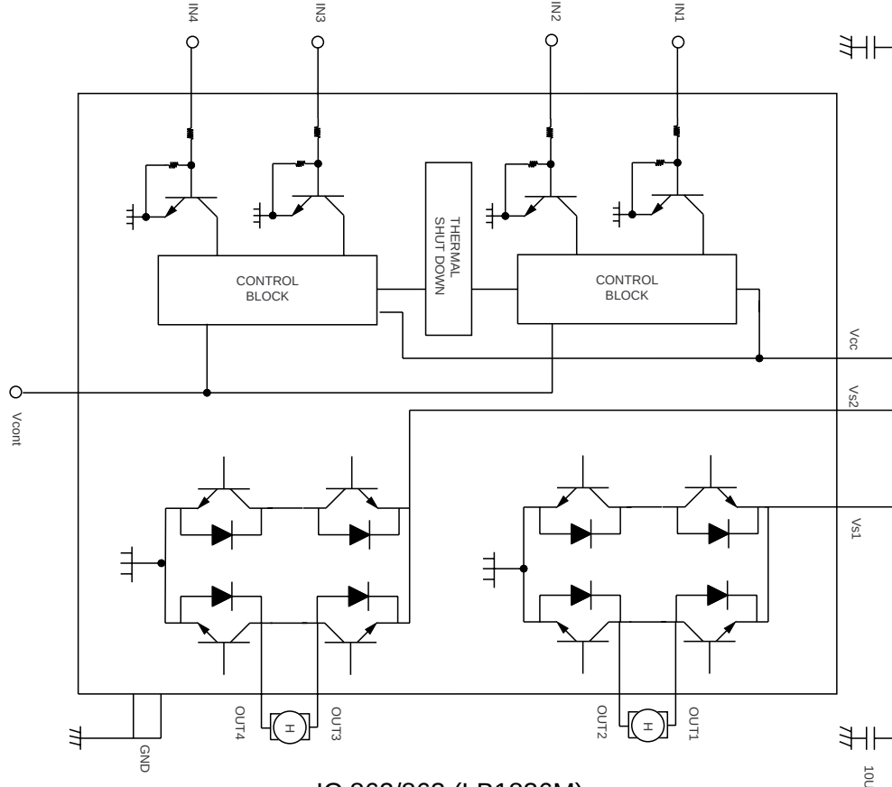
IC 862/863 (LB1836M)
