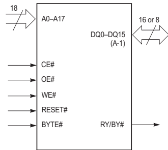
U500 S29AI004D, 4MB Flash Memory IC
