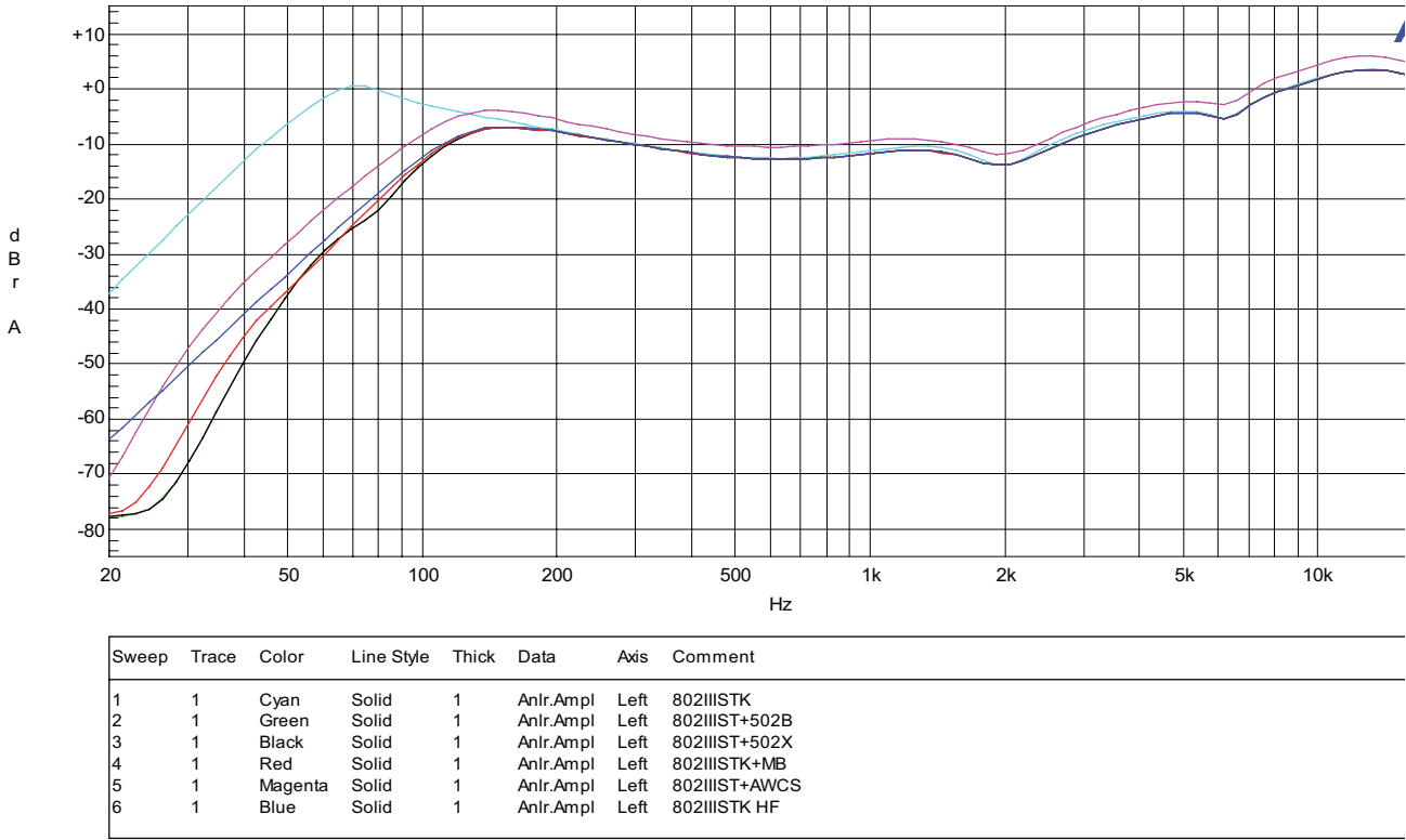
802IIIST CH1, 2
