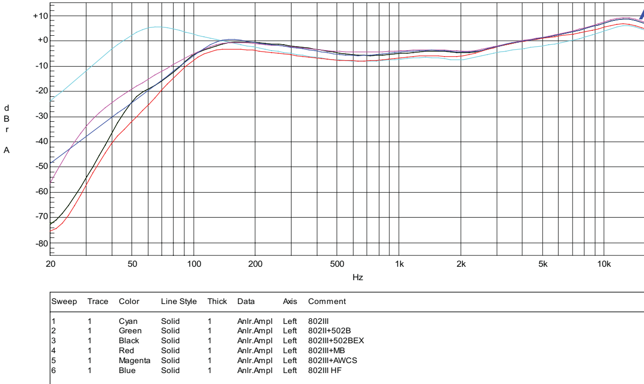
802III CH1, 2
