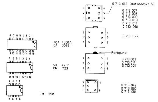
Integrierte Schaltungen integrated circuits
