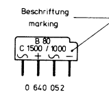
Gleichrichter rectifiers
