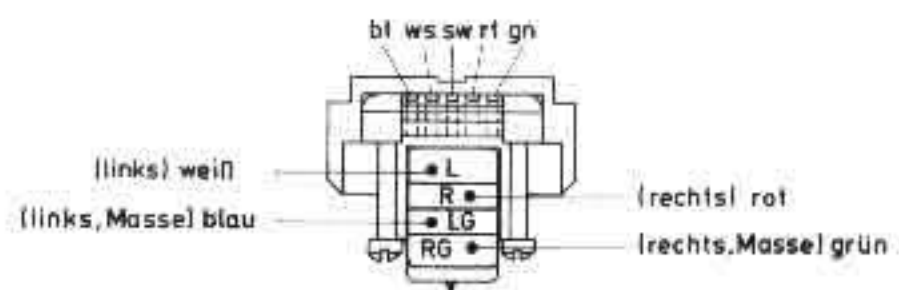
Systemanschluss
