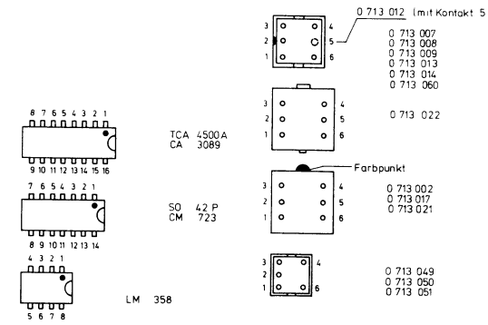
Integrierte Schaltungen integrated circuits
