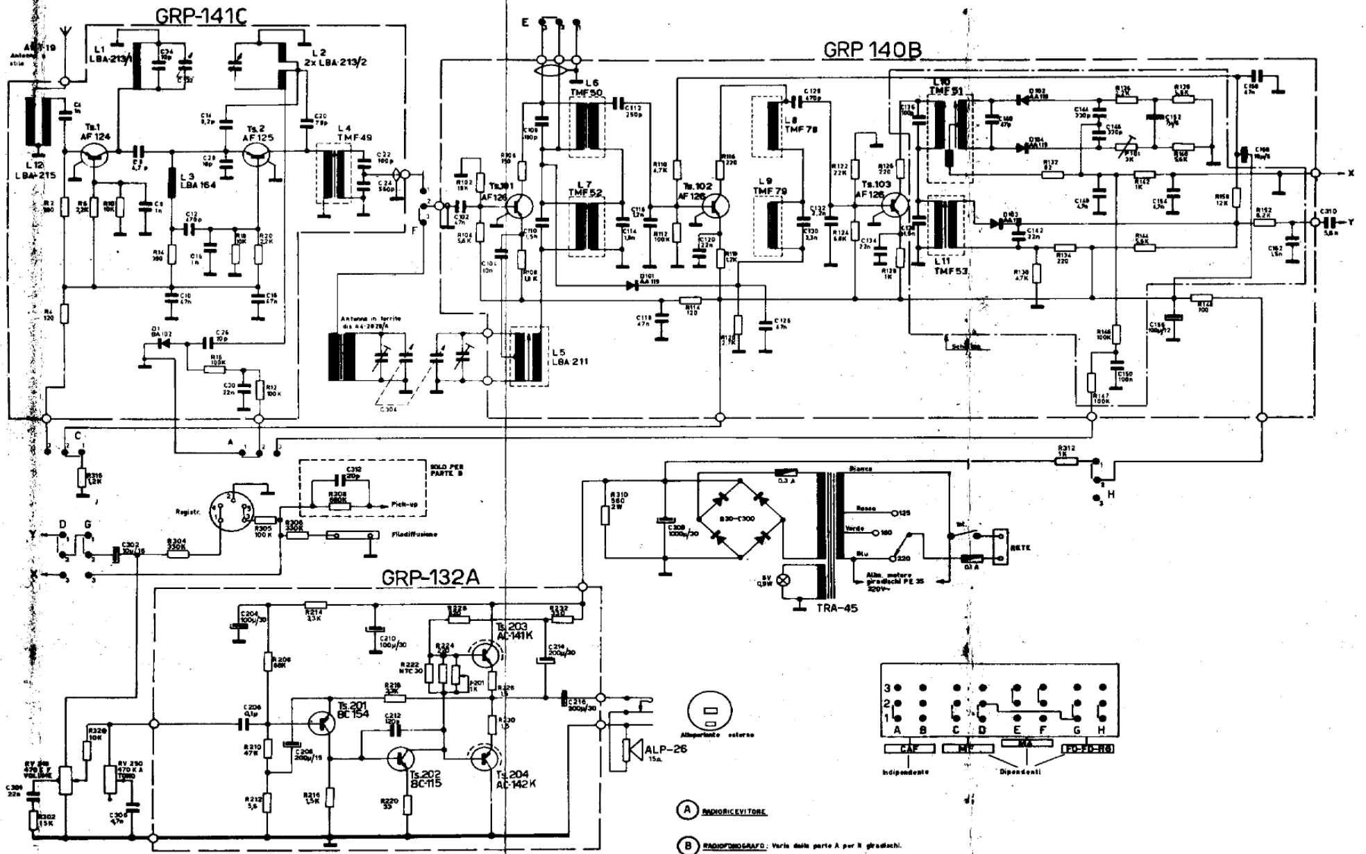
Tavola H — Schema di apparecchio AM/FM a nove transistor e cinque diodi. Il commutatore è in posizione « radio OM » (AM = modulazione di ampiezza) (Brionvega mod. RR-128).
