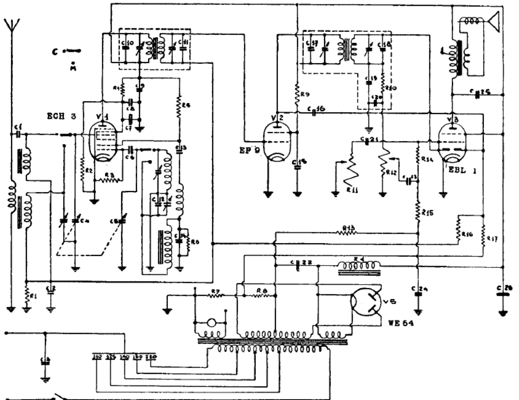
RADIO CARISCH. — Mod. « Emilia e Sicilia ». — Produzione 1940-1941. — Media frequenza: 465 kHz.
