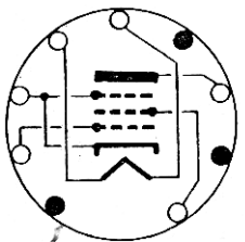
EL84
