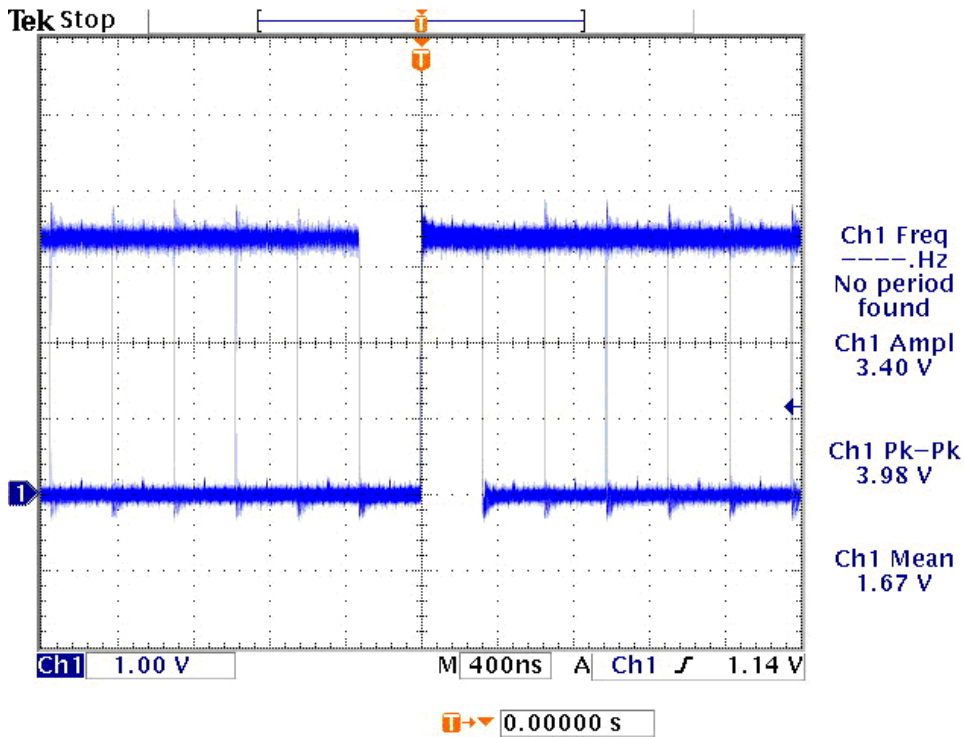
(AUDIO SDAT0) U16:CS4360 Pin2
