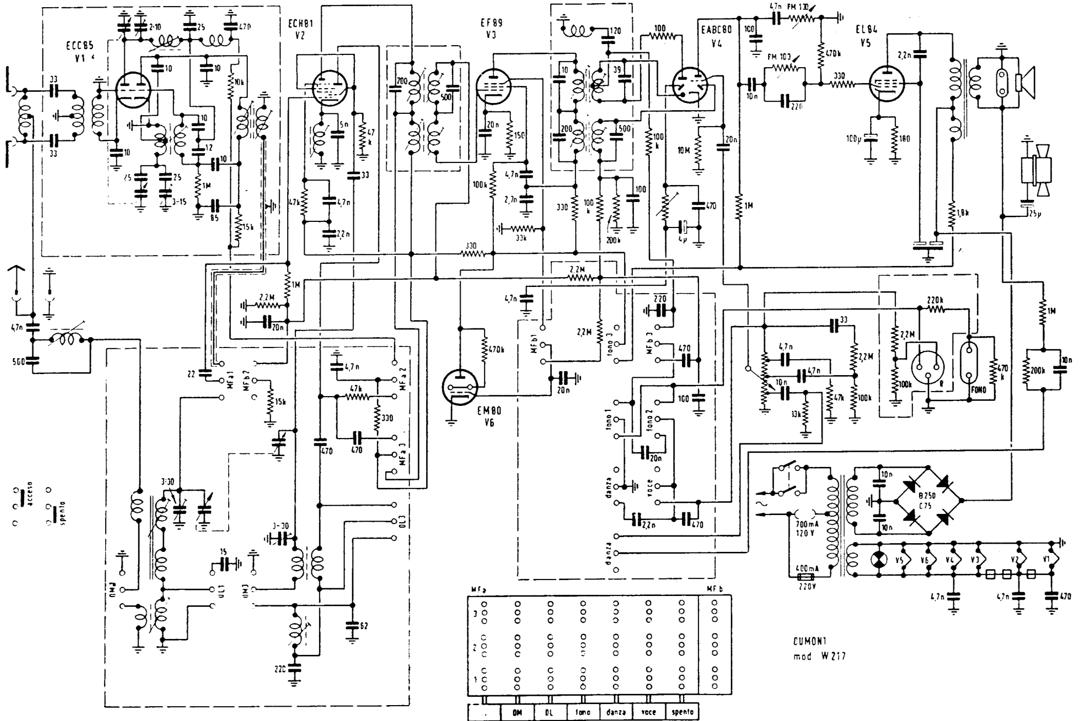
Schema elettrico del radiorecettore Dumont, mod. W 217
