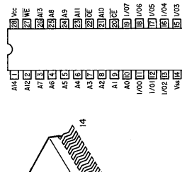
HM65256BLFP-10 (SU: IC705)
