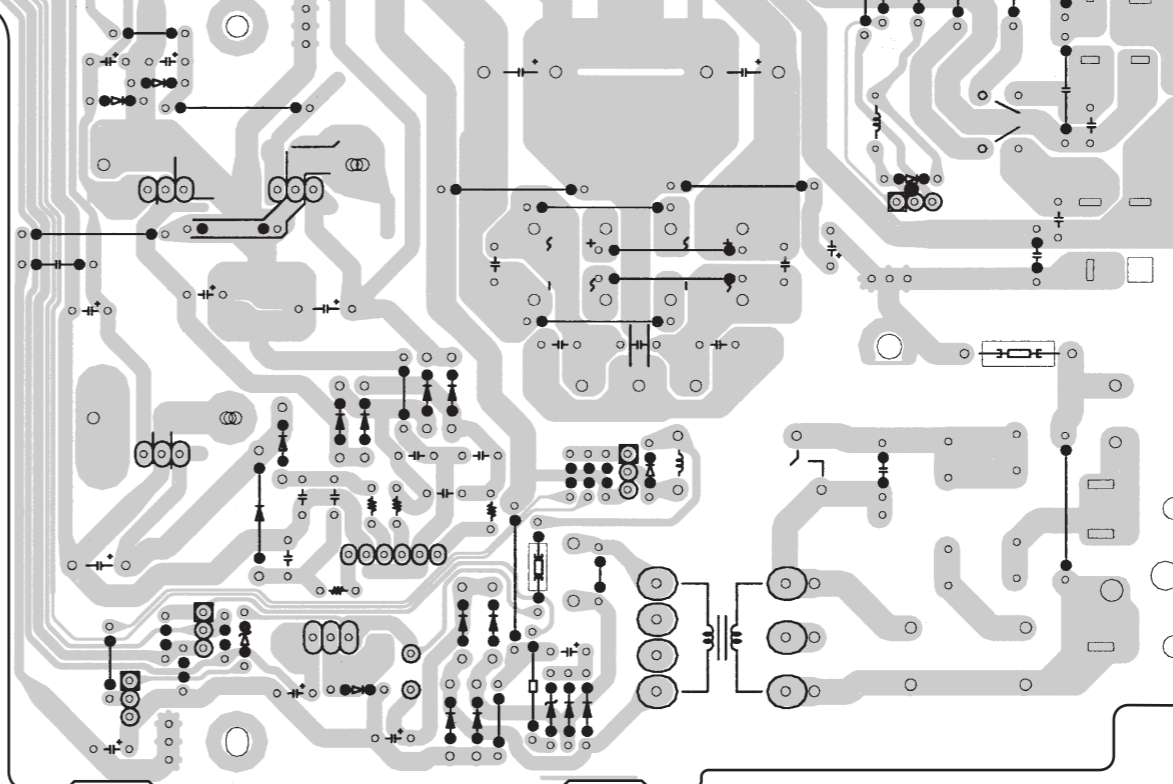
MAIN P.W.B.
