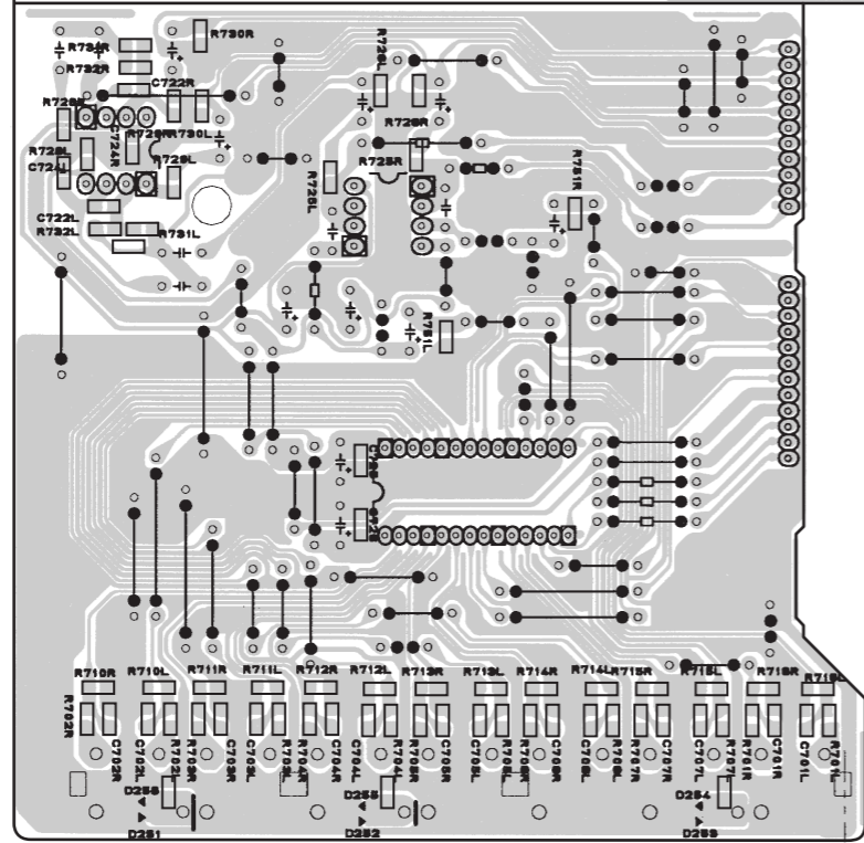
INPUT P.W.B.
