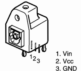
GP1F32T (JACK104)
