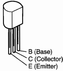
KSA916
