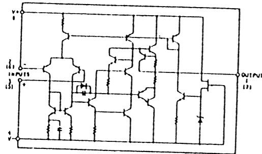
NJM4558D-D
