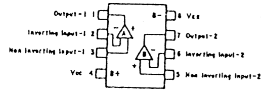
NJM4558D-D
