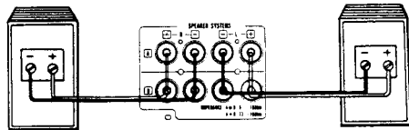
Rechter Lautsprecher Lautsprecherbuchsen Unker Lautsprecher
