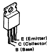
2SA968(Y) 2SC2238(Y)
