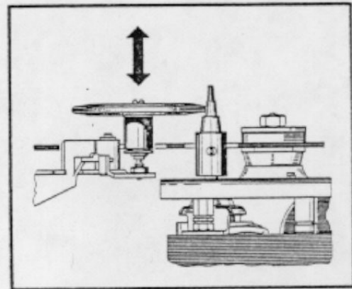
Fig. 5 Stellung der Antriebsrolle (2-Pol-Motor)
