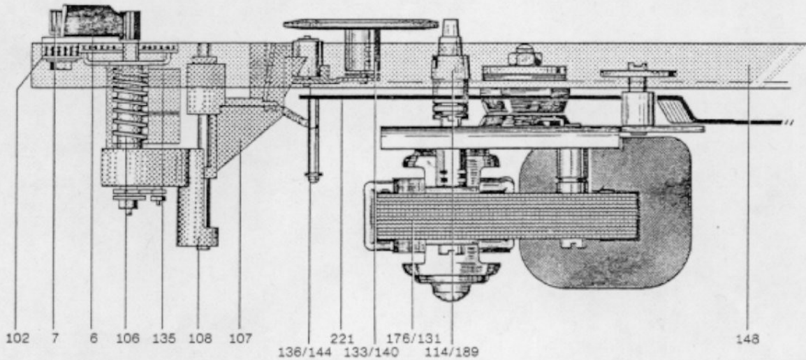
Fig. 2 Motoraufhängung und Antrieb des Plattentellers
