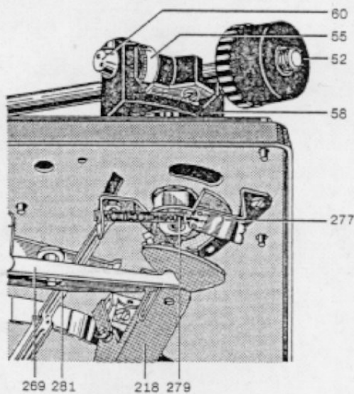
Fig. 8 Tonarmlagerung (Unteransicht)
