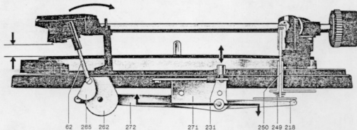
Fig. 11 Tonarmlift (Tonarm abgehoben)
