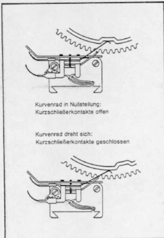
Fig. 14 Kurzschließer
