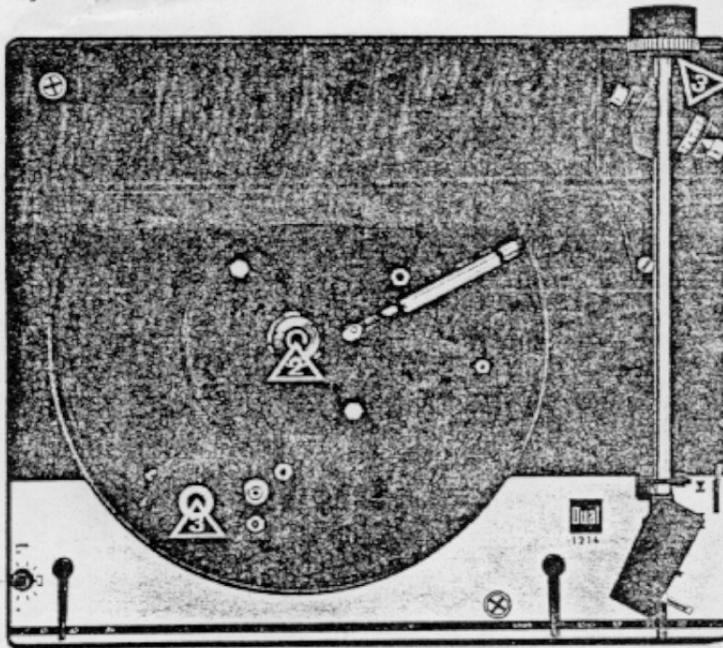
Fig. 26 *,Schmierstellen Über der Platine
