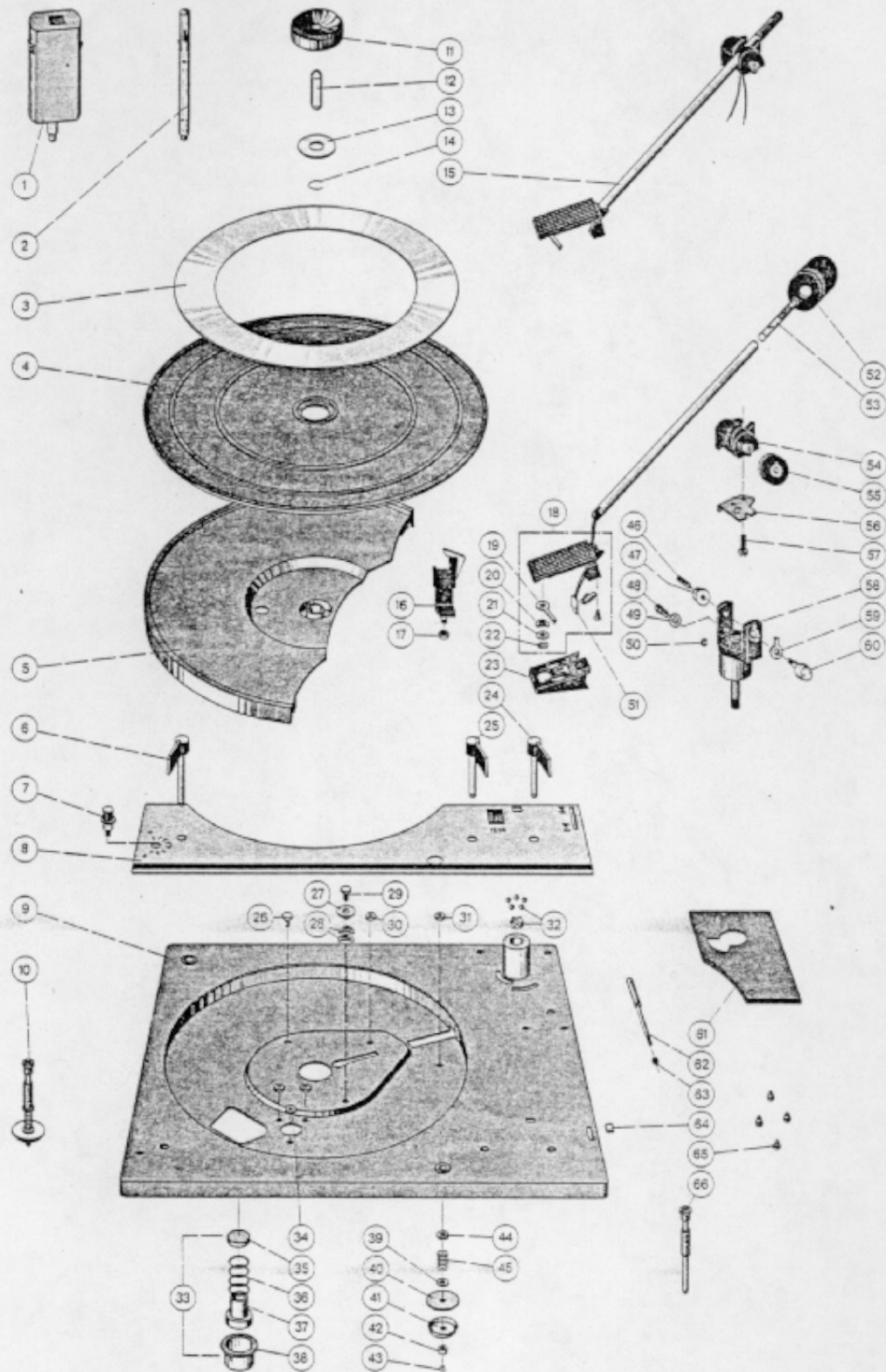
Fig. 24 Explosionsdarstellung, Teile Über der Platina
