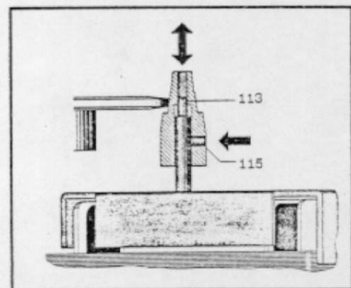
Fig. 6 Stellung der Antriebsrolle (4-Pol-Motor)
