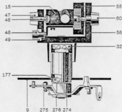
Fig. 7 Tonarmlagerung
