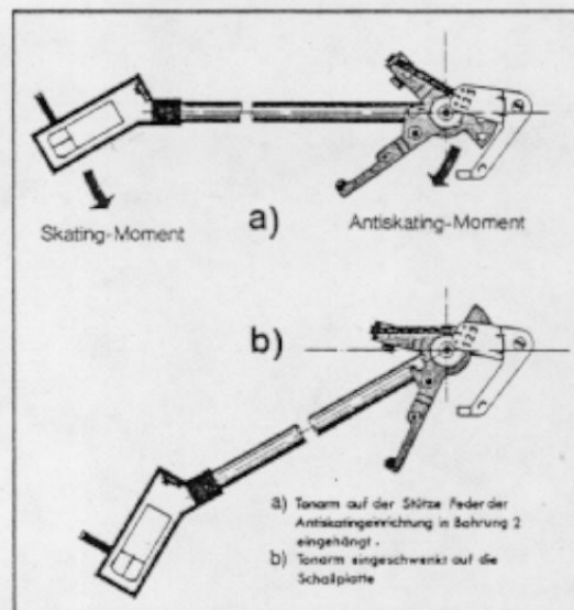
Fig. 9 Antiskatingkraft
