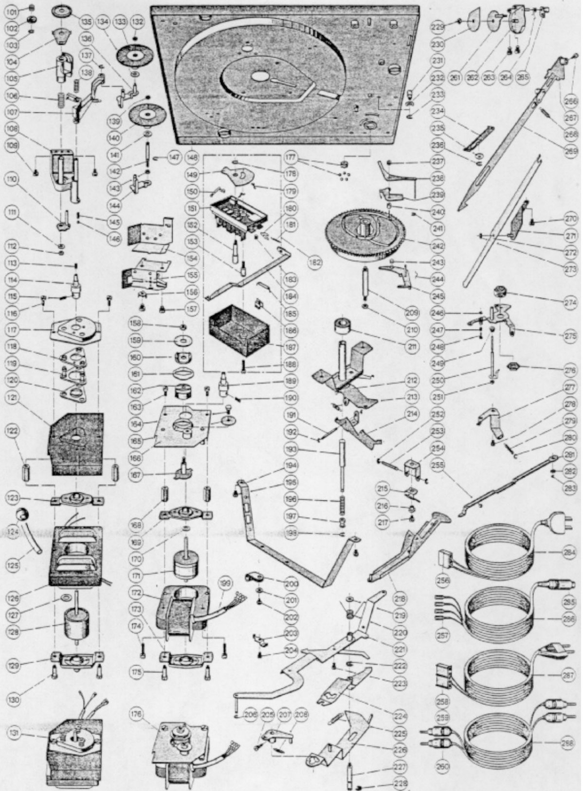
Fig. 25 Explosionsdarstellung, Teile unter der Platine
