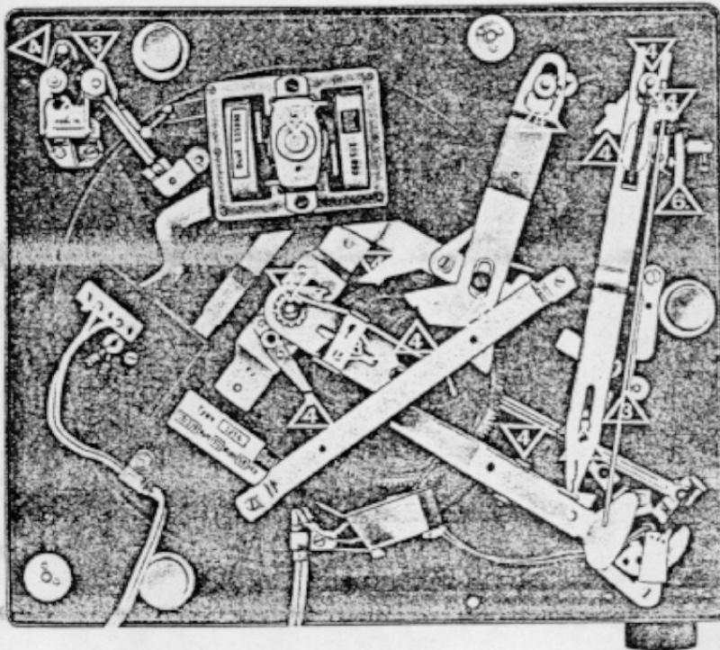
Fig. 27 Schmierstellen unter der Platine
