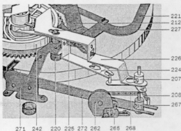
Fig. 12 Startstellung
