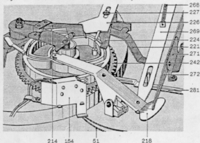
Fig. 10 Kinematik der Tonarmsteuerung
