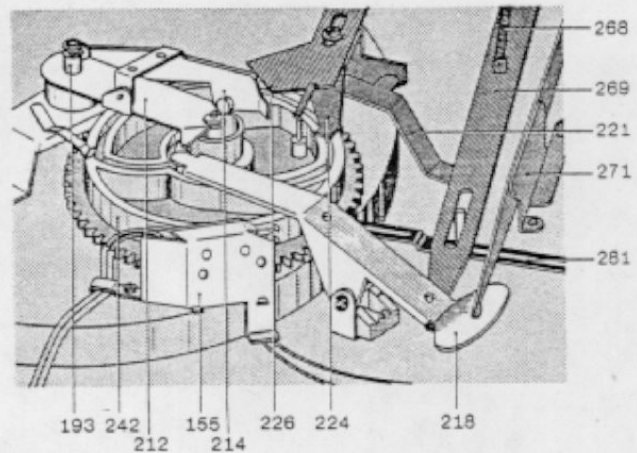
Fig. 15 Schallplattenabwurf
