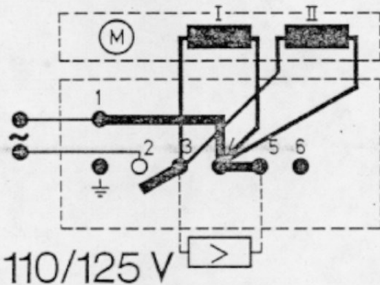
Fig. 3 Anschluß der Feldspulen (ohne Spannungszähler)
