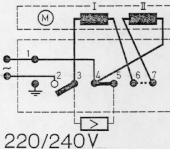
Fig. 4 Anschluß der Feldspulen (mit Spannungszähler)
