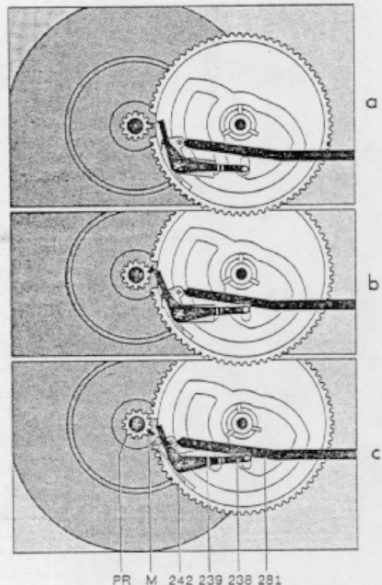
Fig. 16 Einleitung der Wechsel- bzw. Abstellfunktion
