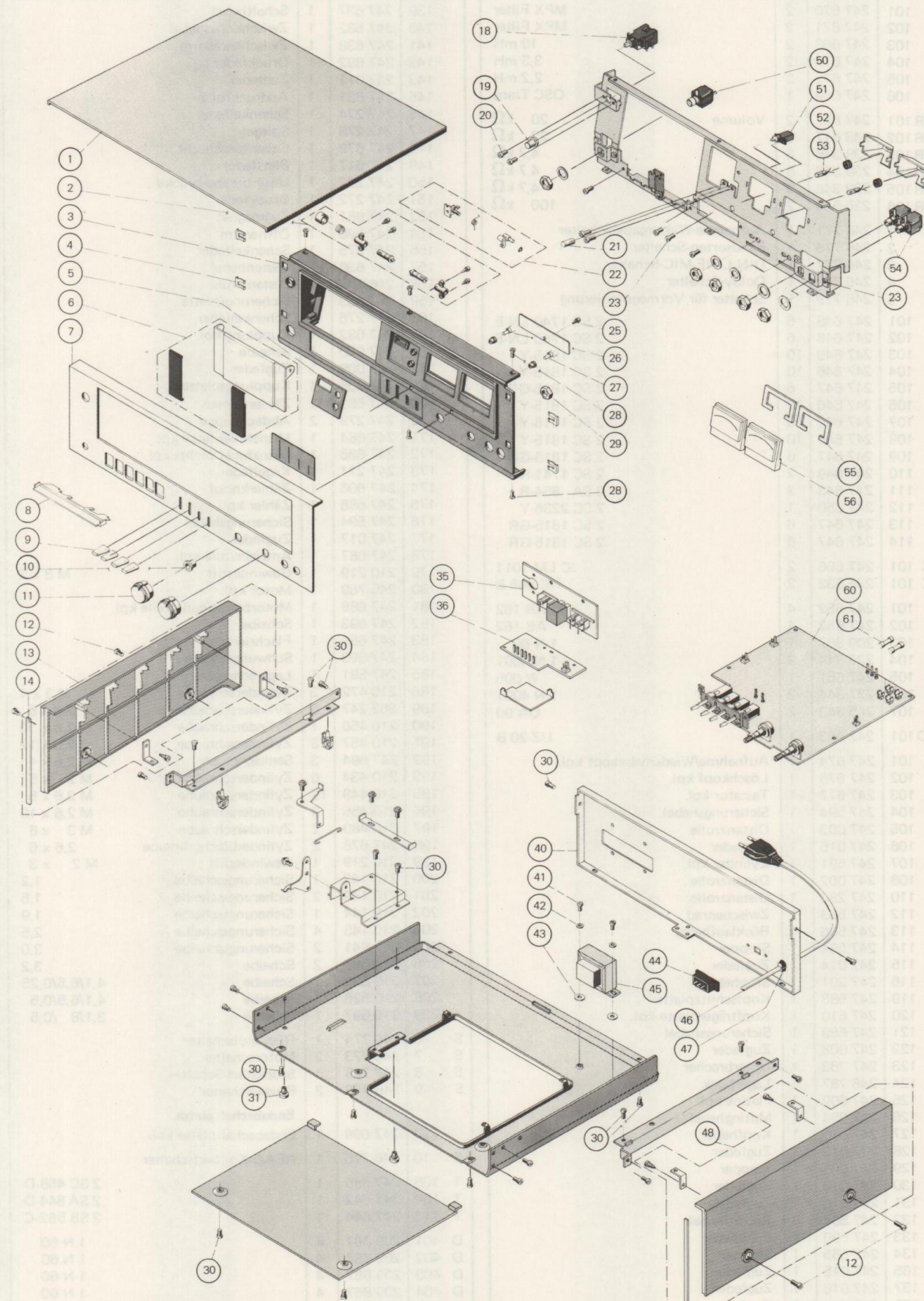
Fig. 11 Explosionsdarstellung 1
