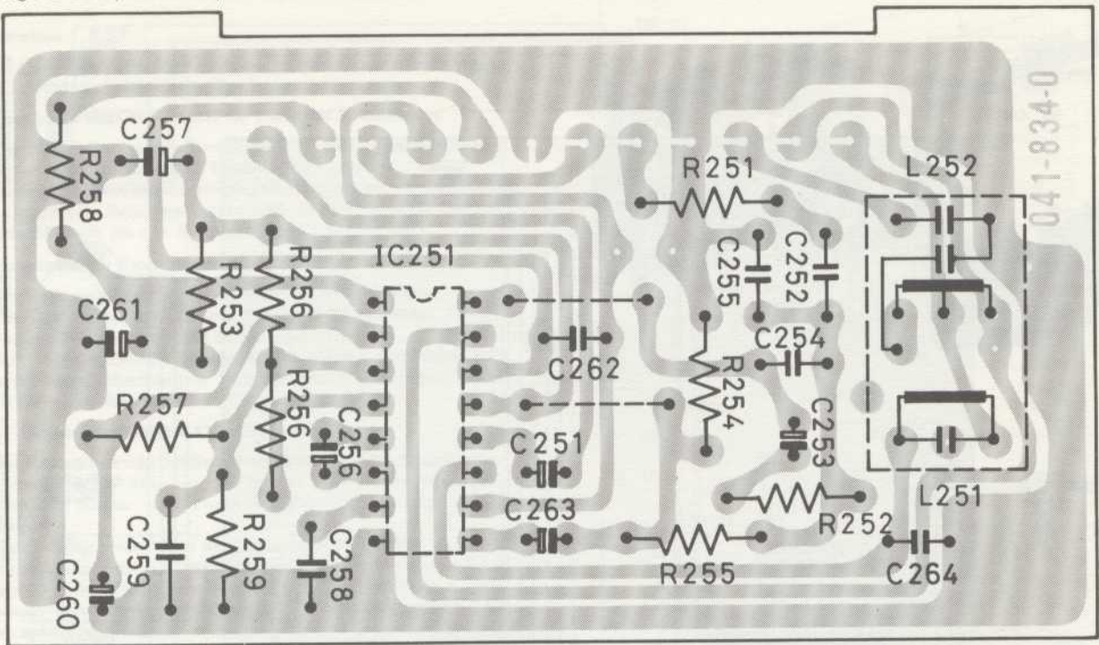
Fig. 10 Dolby-Verstärkerplatte 264 107 (Leiterseite)
