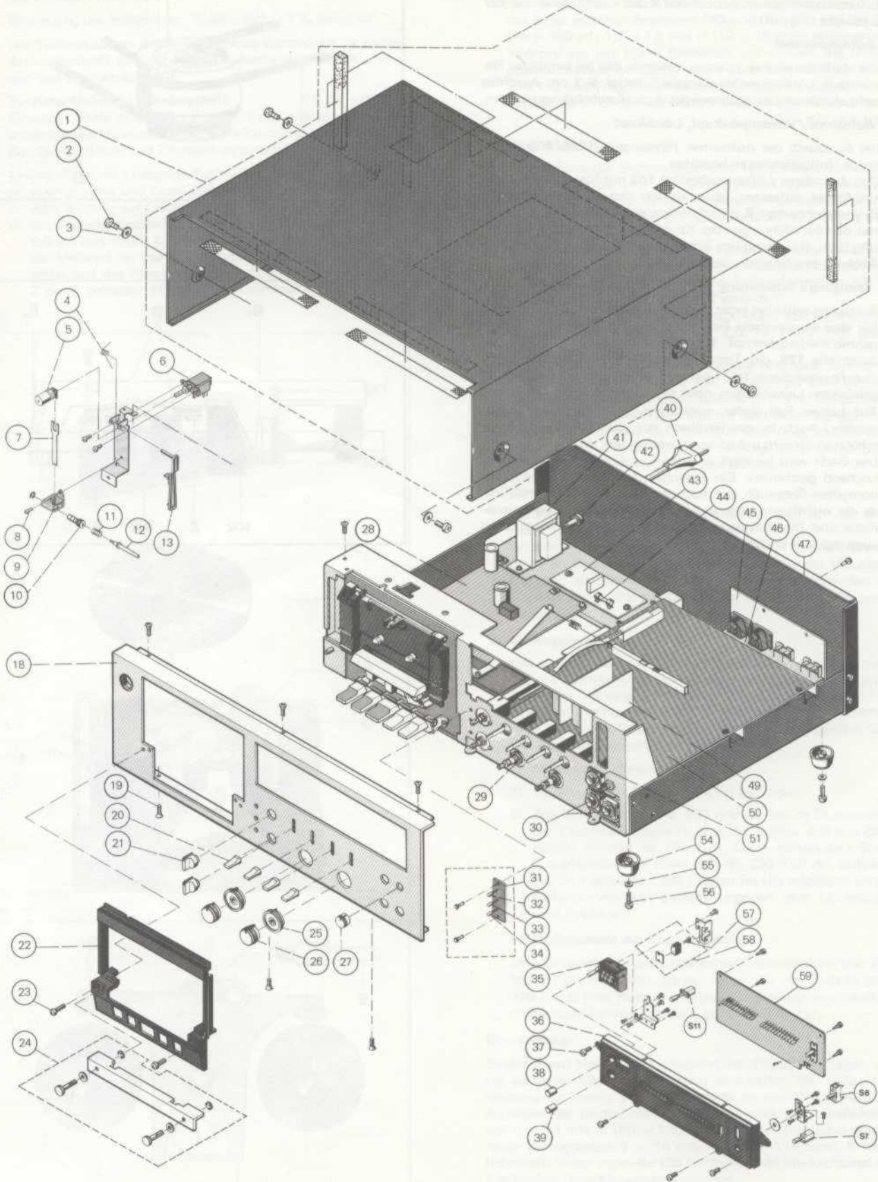
Fig. 21 Explosionsdarstellung 1
