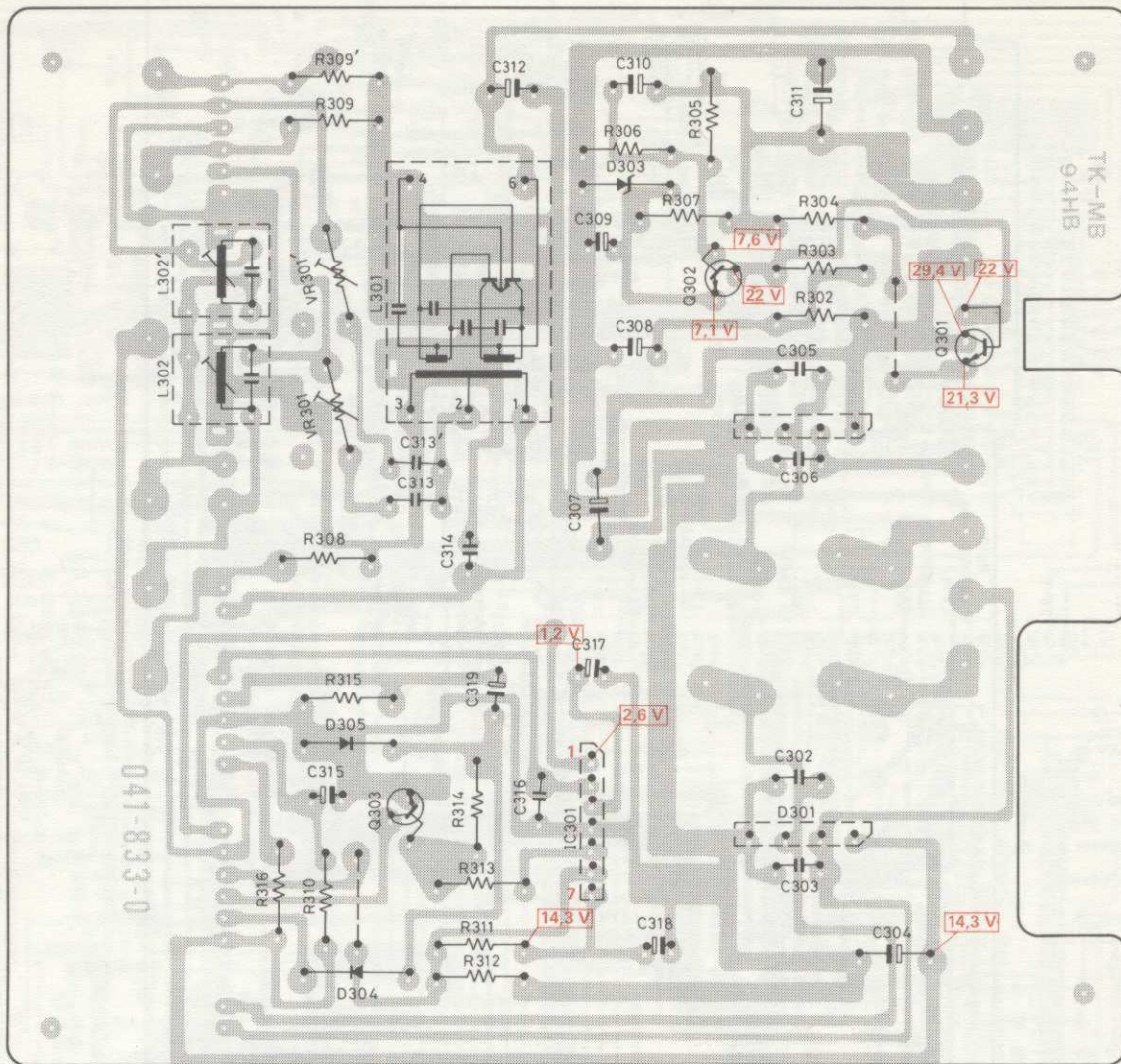
Fig. 8 Oszillatorplatte 264 097 (Leiterseite)
