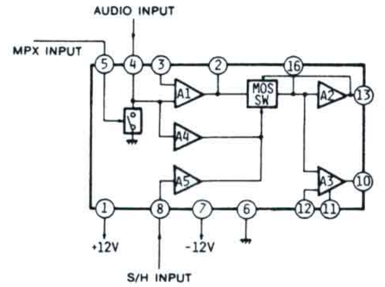
IC501L, R(HA12053)
