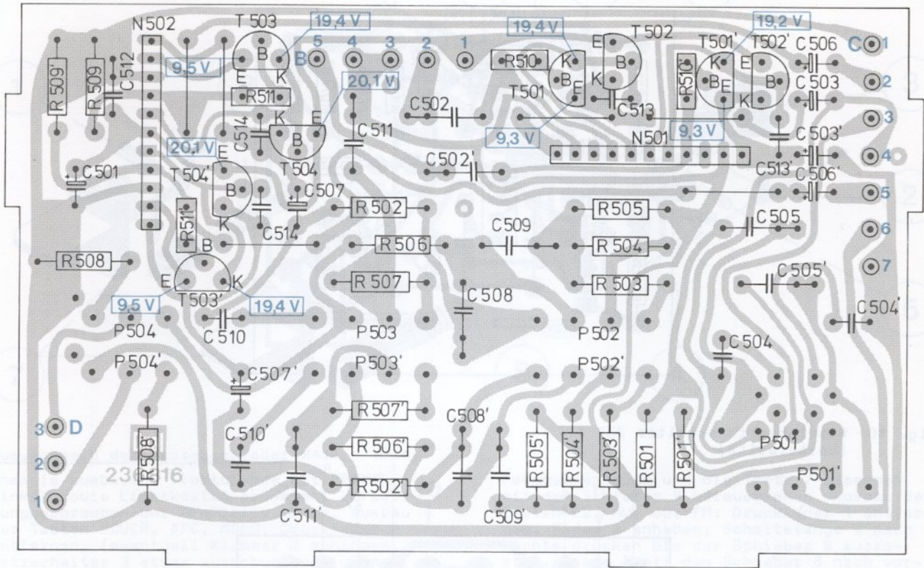
Fig. 7 Regelverstärker 239 179 (Leiterseite)
