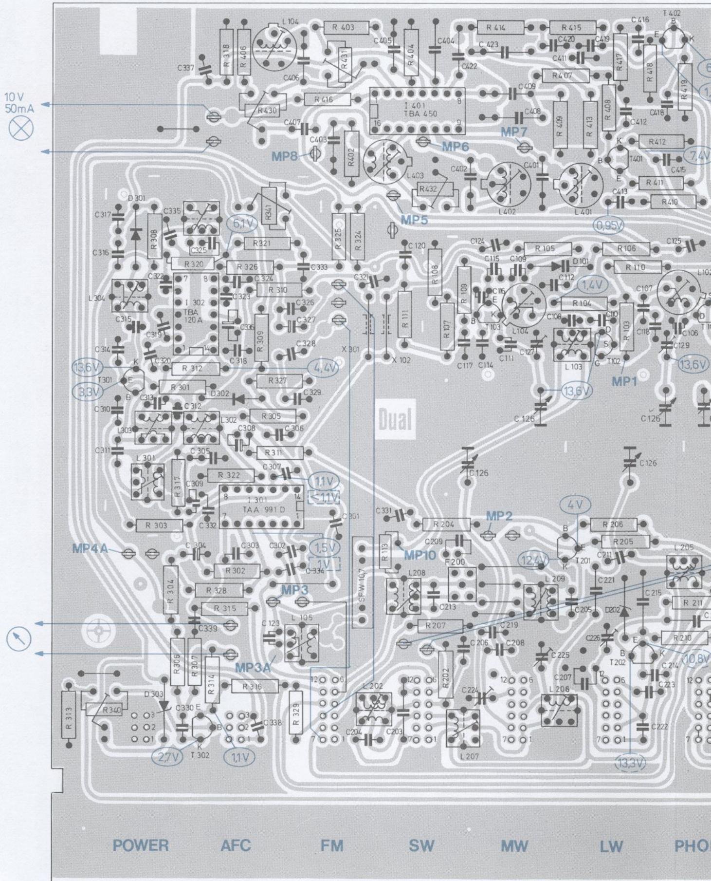
Fig. 4 HF-Platte 231 254
