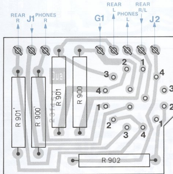
Fig. 10 Betriebsartenschalter 239 177 (Leiterseite)
