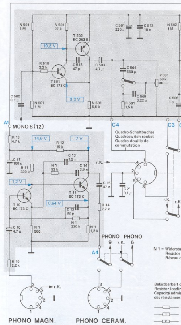
Fig. 3 Schaltbild NF
