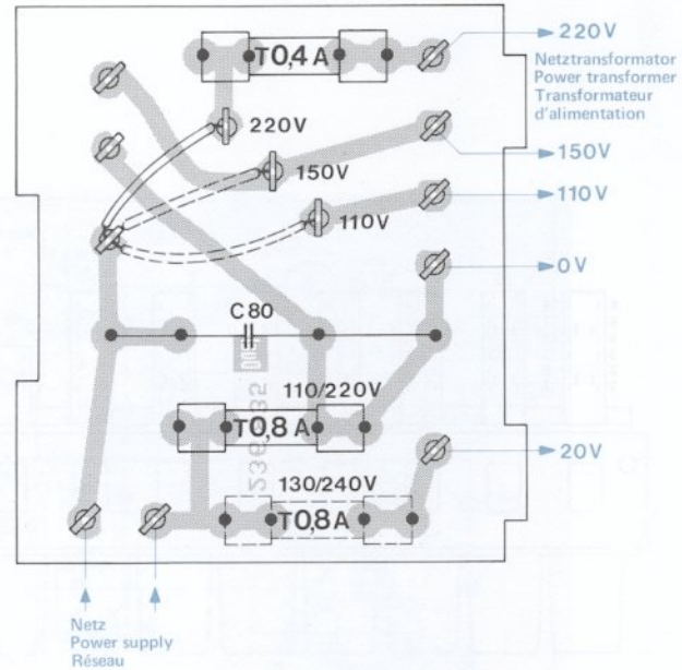
Fig. 5 Netzanschlußplatte 236 834 (Bestückungsseite)
