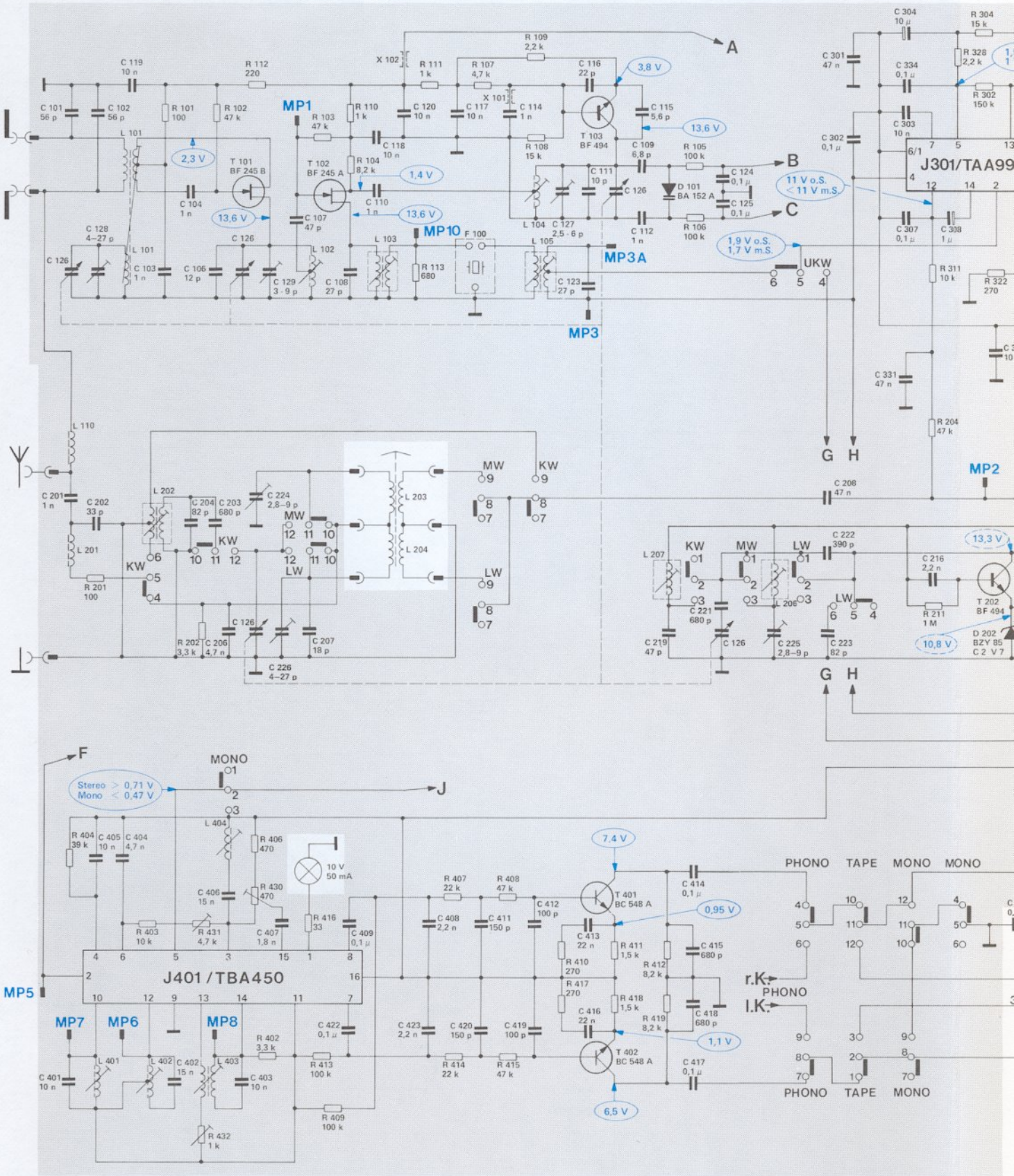
Fig. 2 Schaltbild HF
