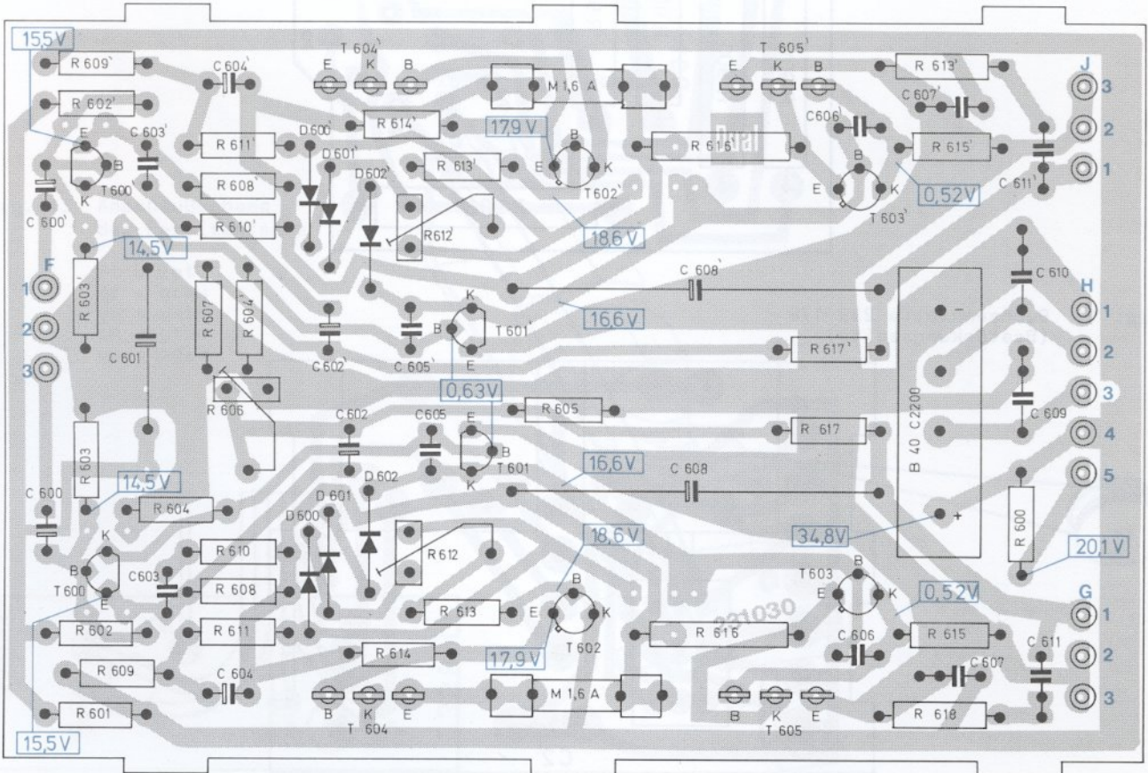
Fig. 8 Endverstärker 234 147 (Leiterseite)
