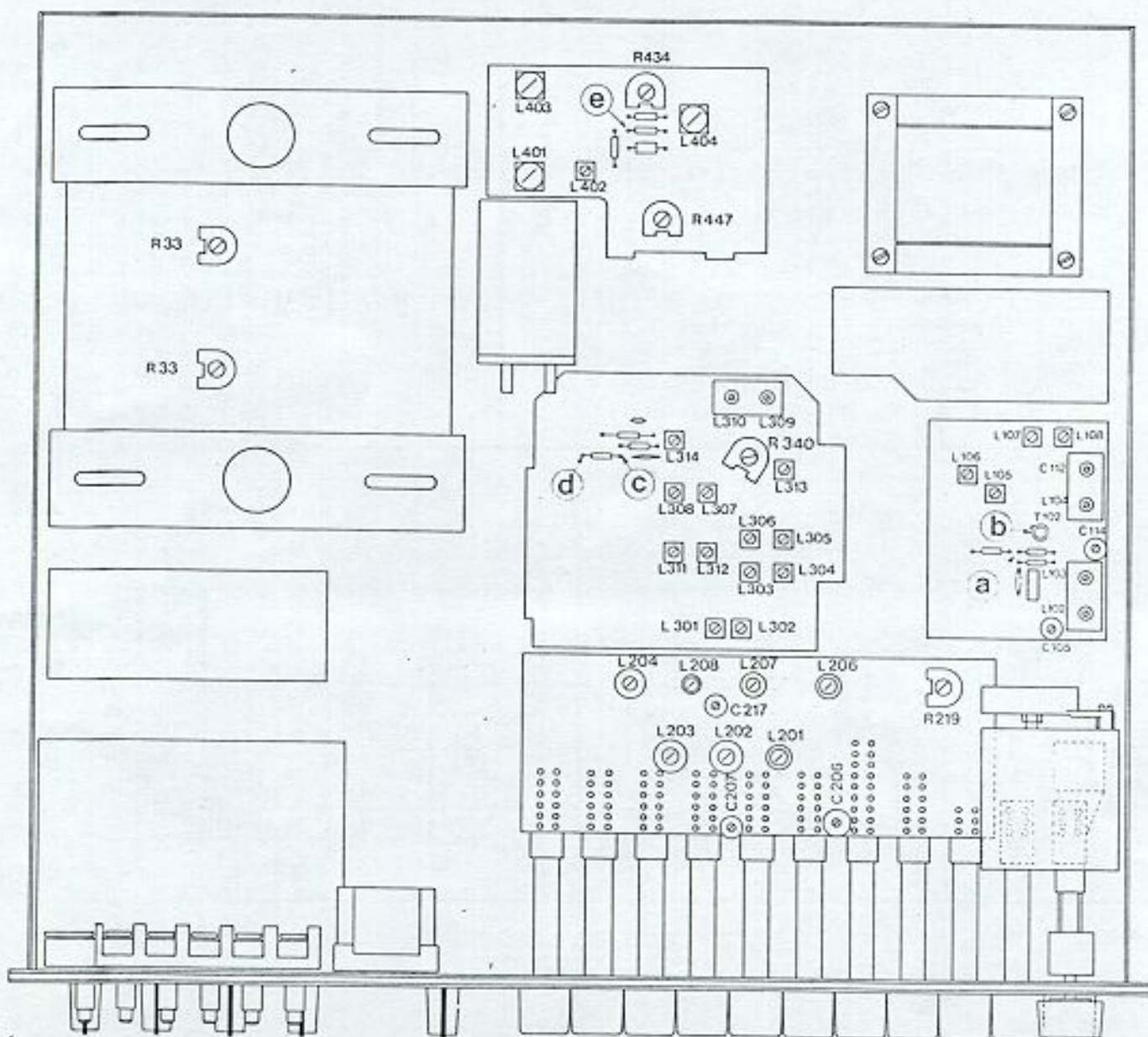
Fig. 1 Abgleichpositionen
