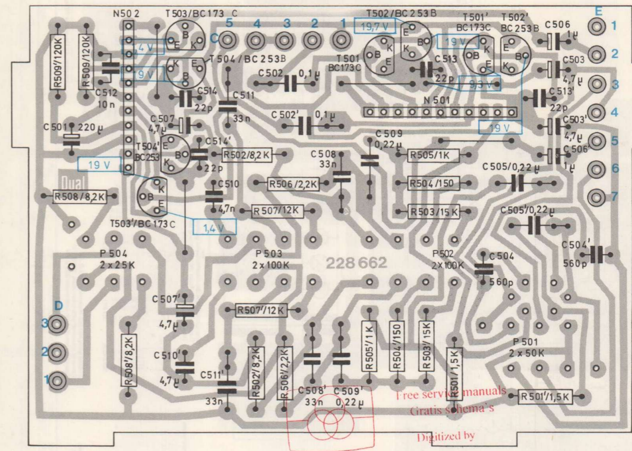
Fig. 9 Regelverstärker 230 606 (Leiterseite)
