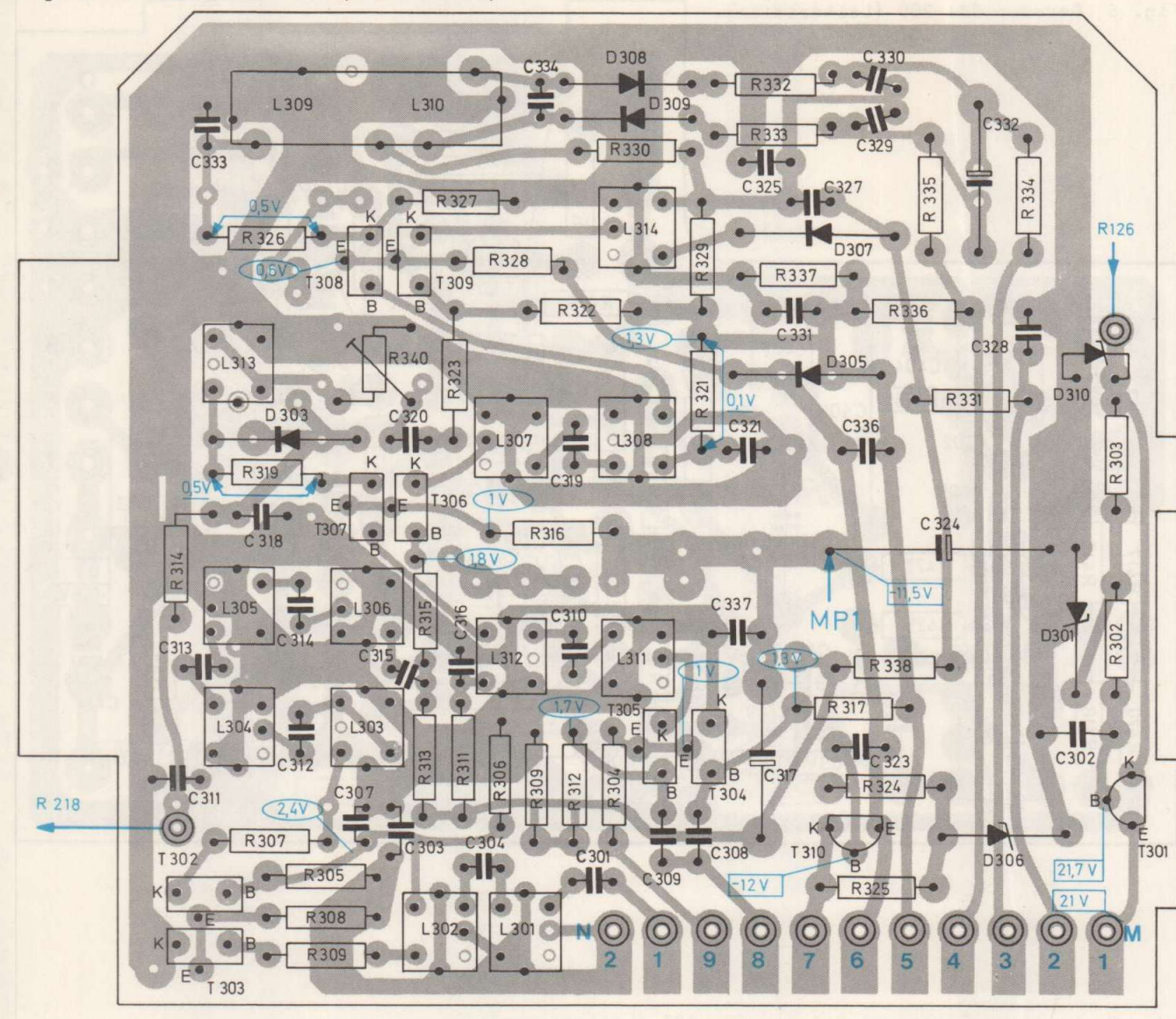
Fig. 4 ZF-Platte 231 220 (Leiterseite)
