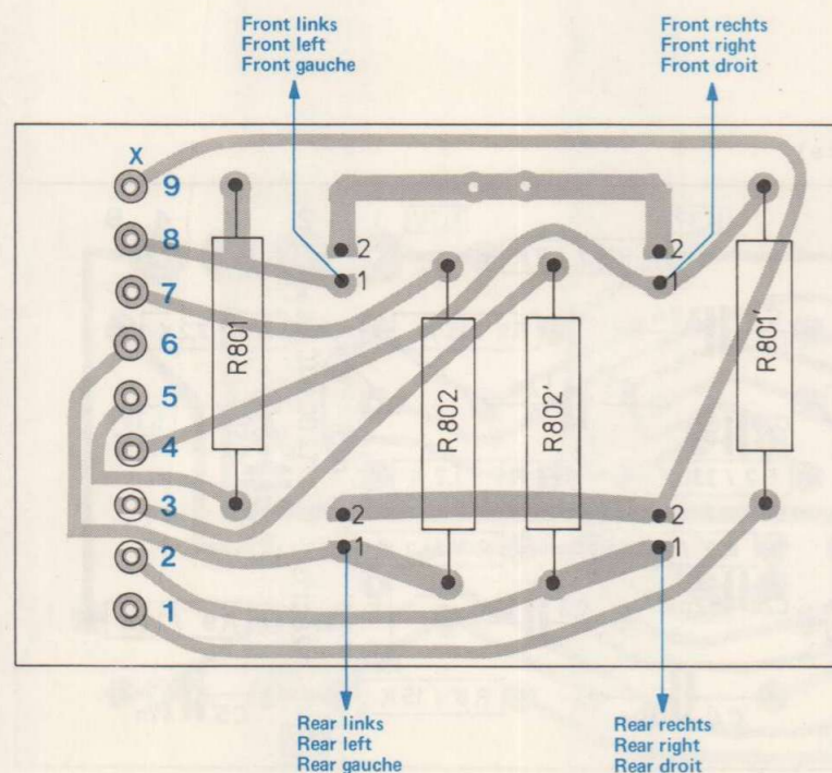
Fig. 7 Lautsprecheranschlußplatte 234 475 (Leiterseite)
