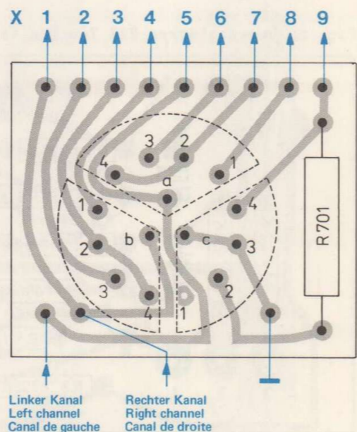
Fig. 8 Betriebsartenschalterplatte 234 473 (Leiterseite)
