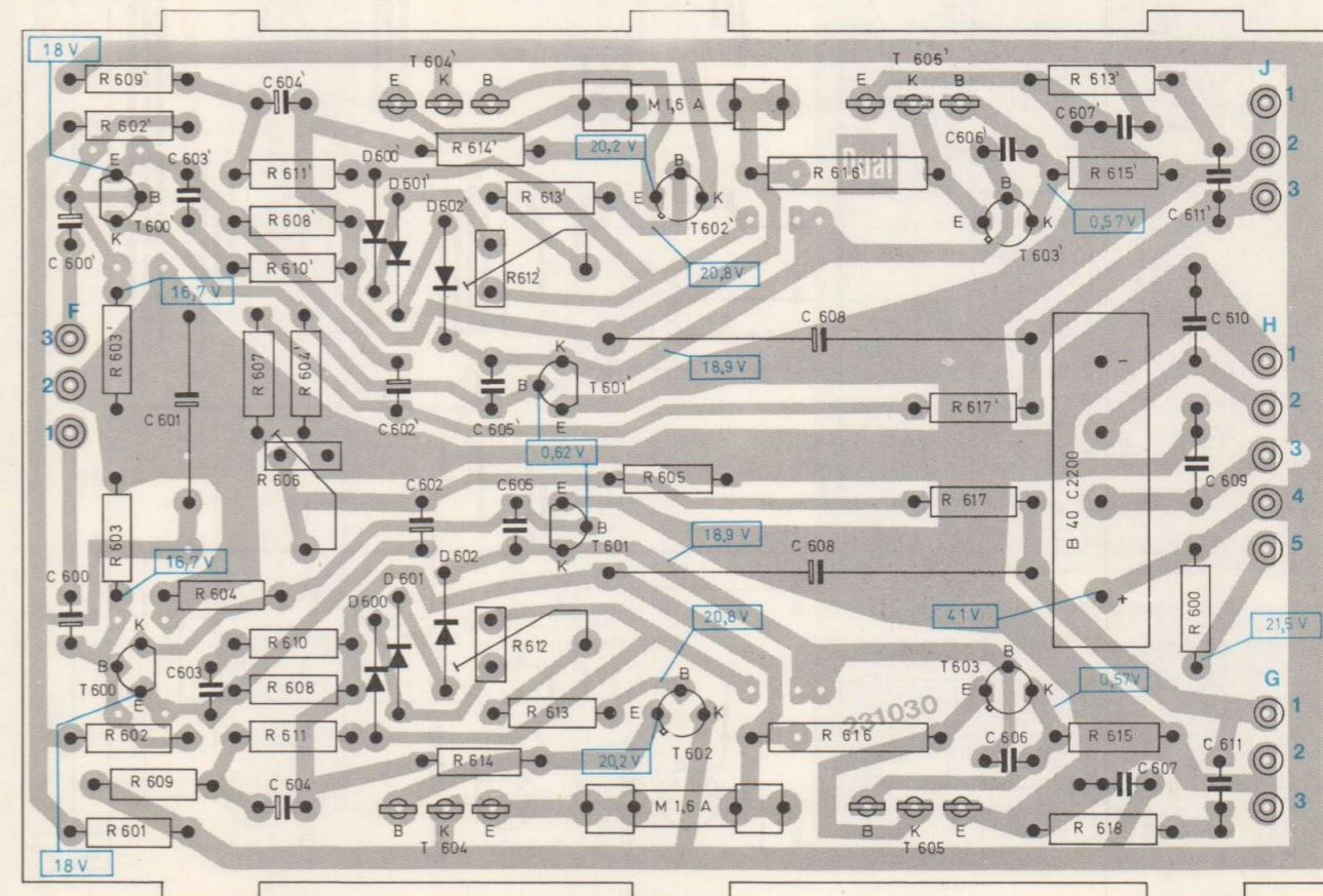
Fig. 10 Endverstärker 234 147 (Leiterseite)
