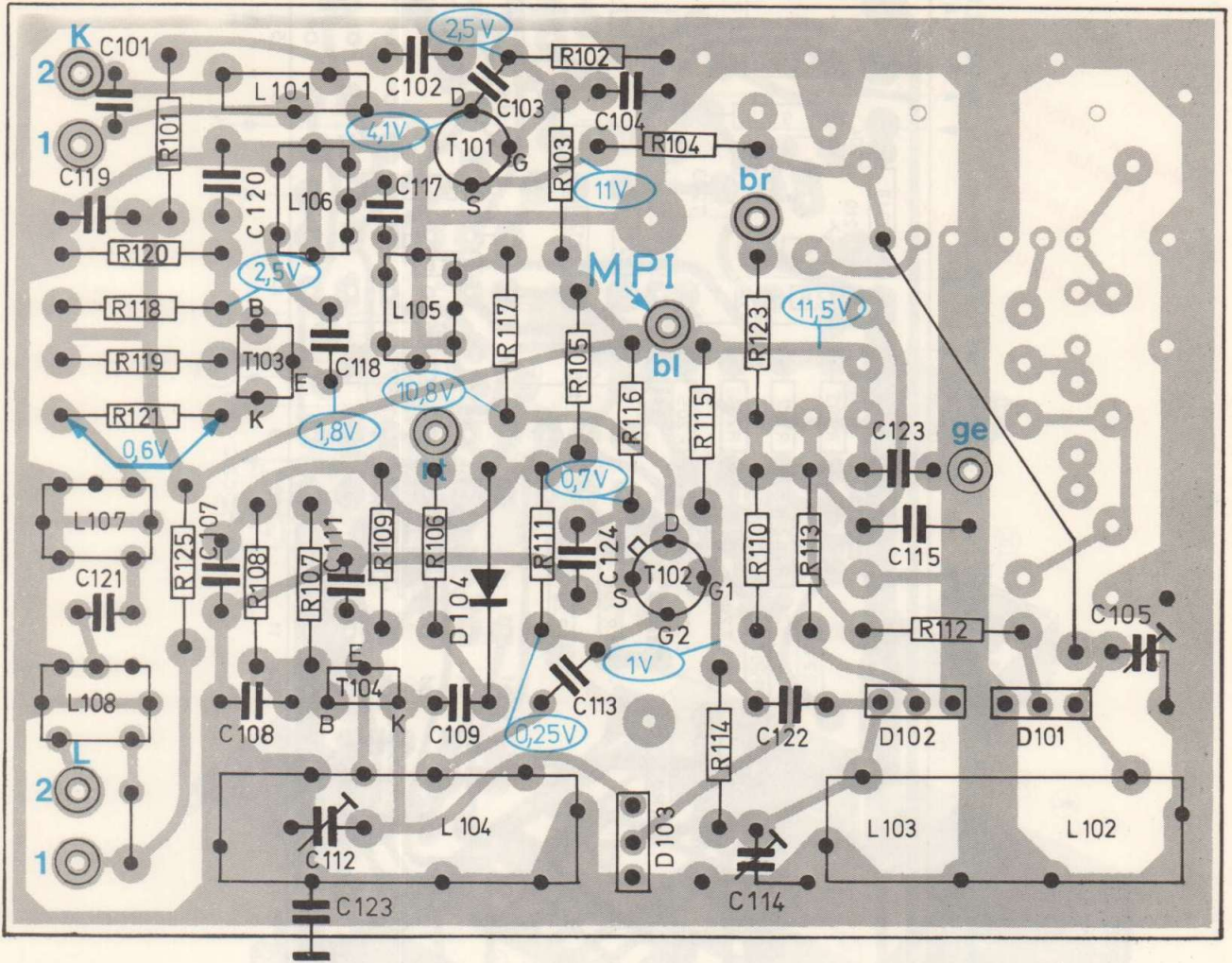
Fig. 11 UKW-Teil 231 211 (Leiterseite)
