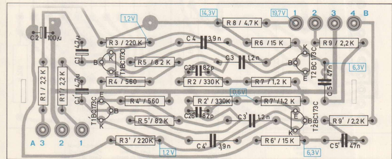
Fig. 5 Vorverstärker 227 746 (Leiterseite)
