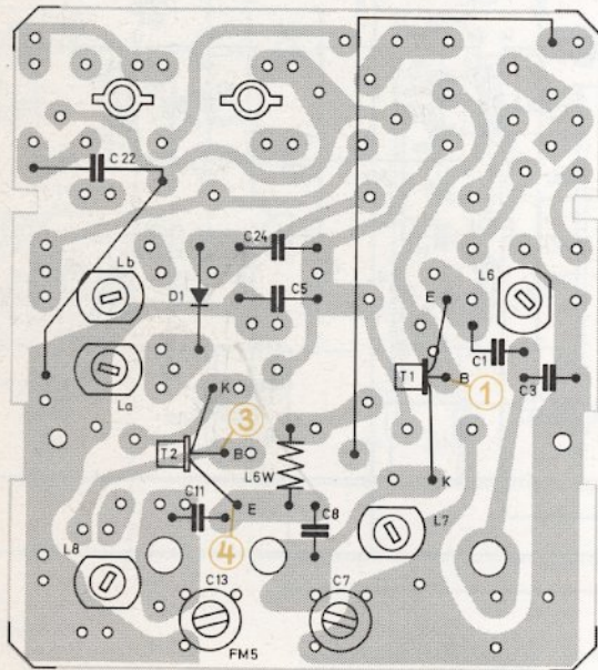
Fig. 8 UKW-Platte (Spulenseite)
