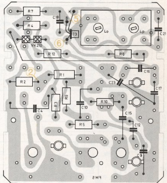
Fig. 9 UKW-Platte (Bestückungsseite)
