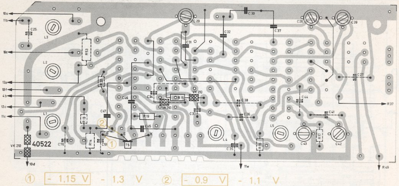
Fig. 7 Tastenschalter-Platte
