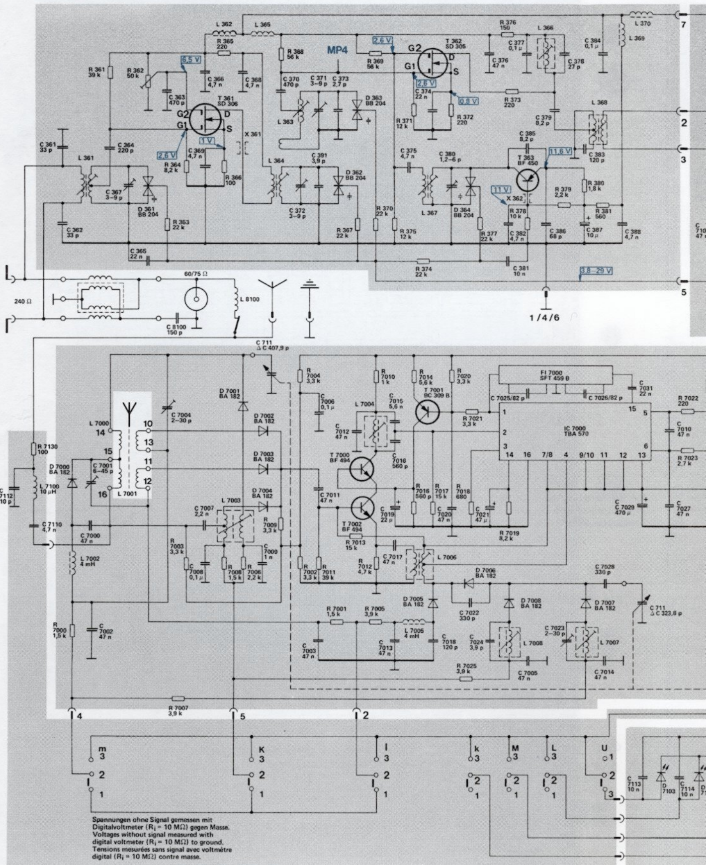
Fig. 2 Schaltbild
