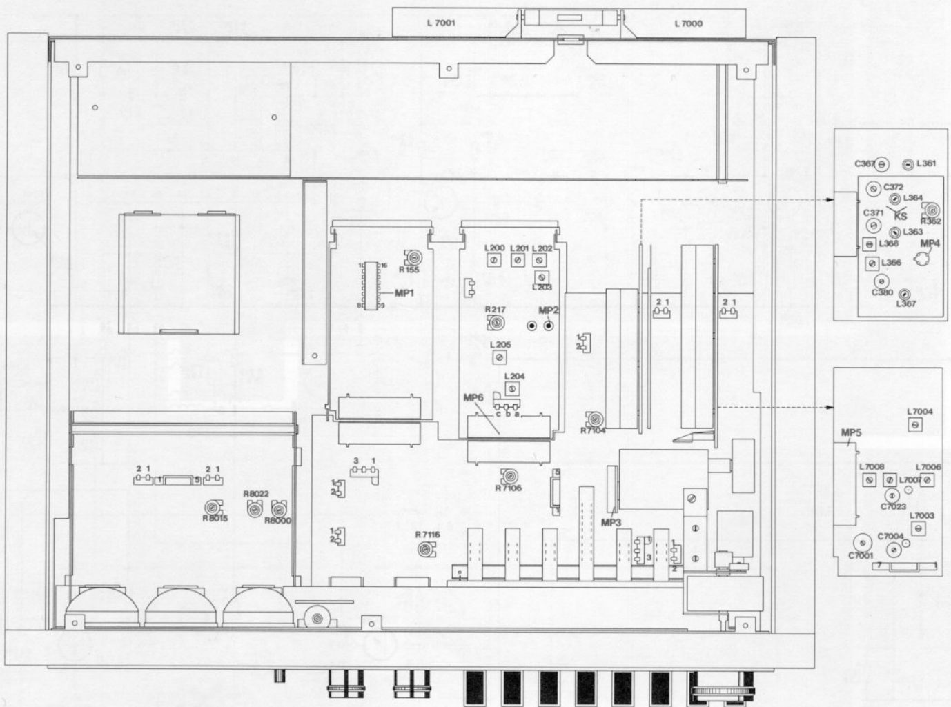
Fig. 1 Abgleichpositionen
