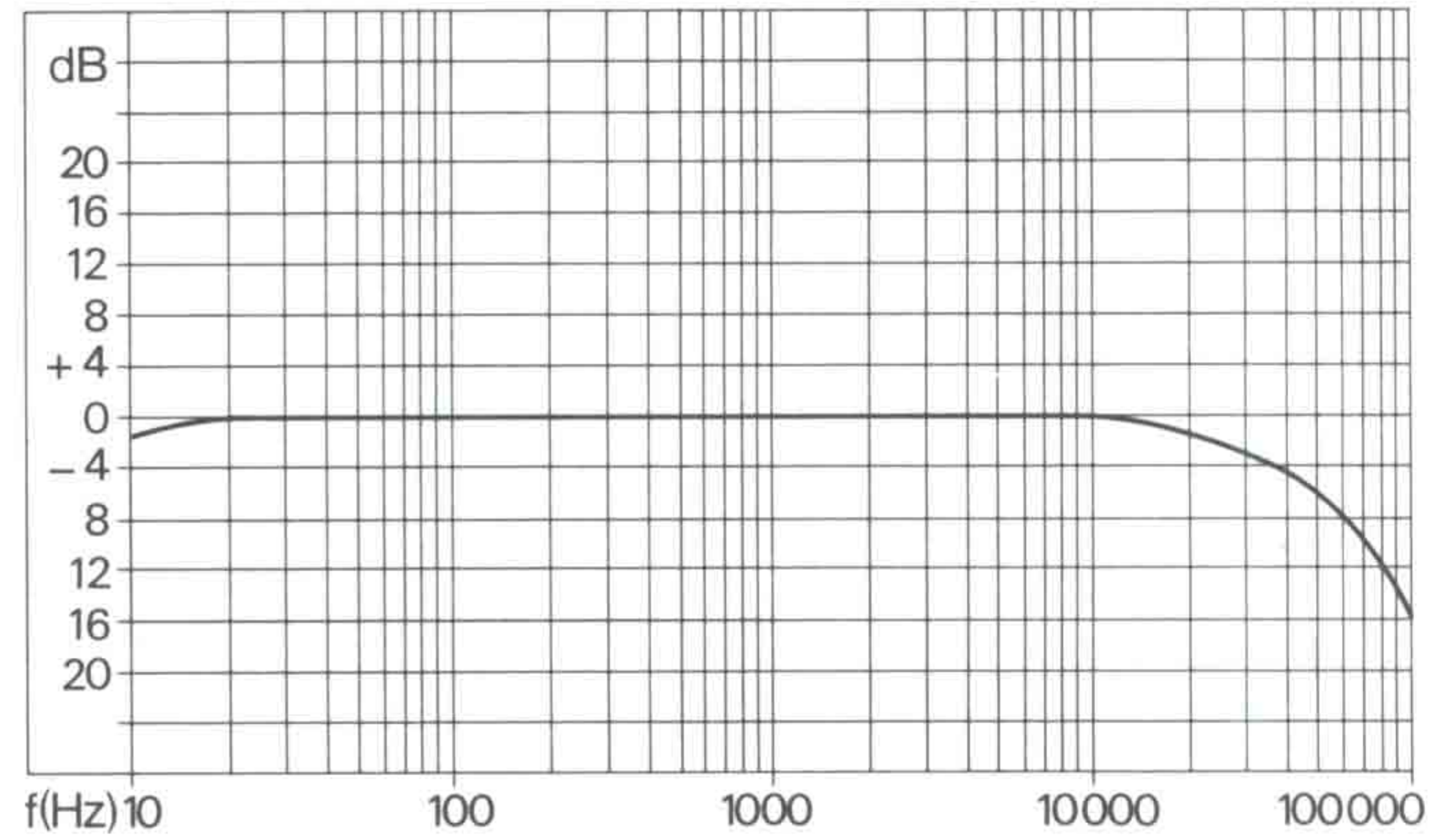
Fig. 2 Frequenzgang des Mikro-Vorverstärkers
