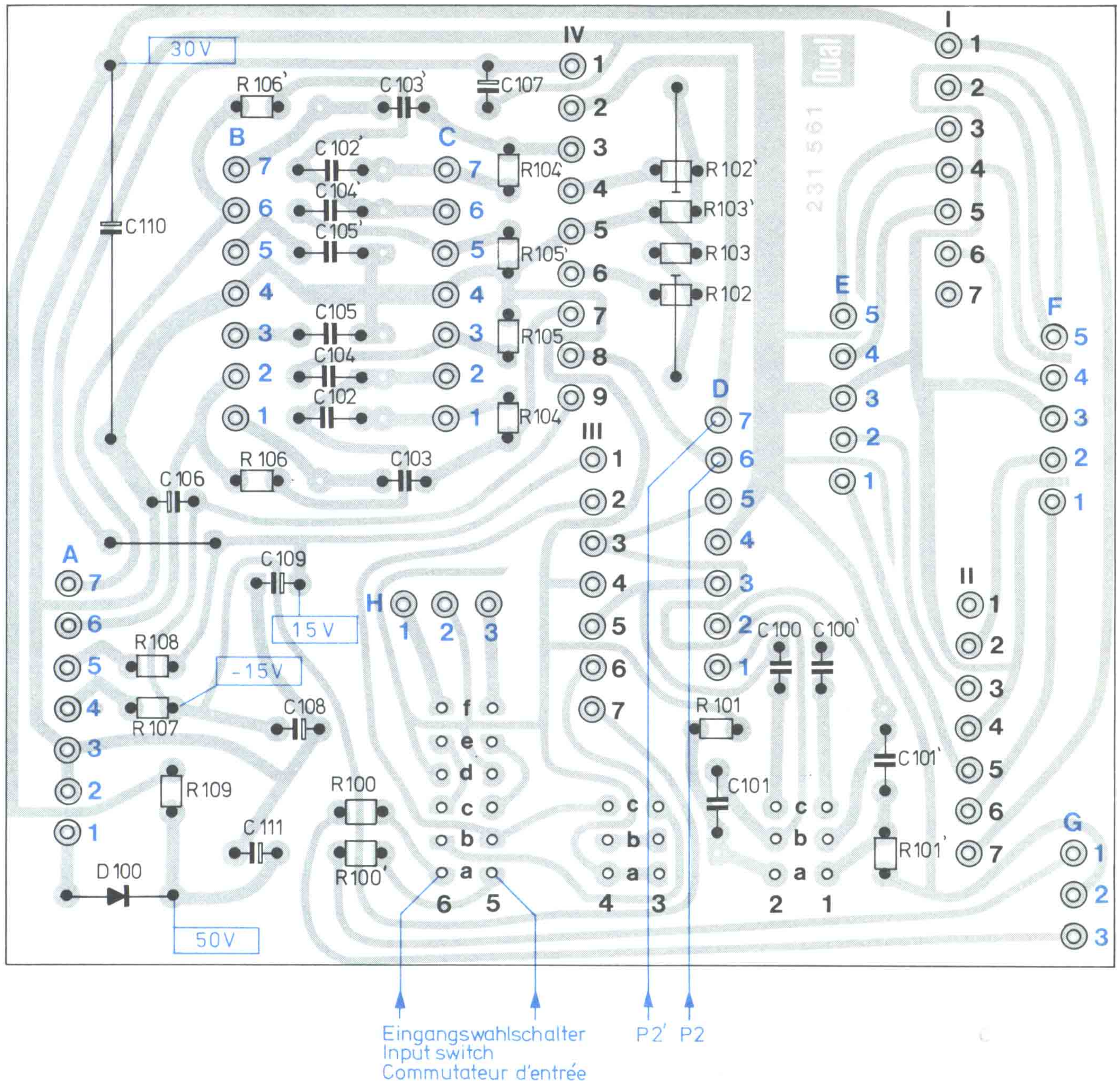
Fig. 8 Steuerverstärker 233 988 (Leiterseite)
