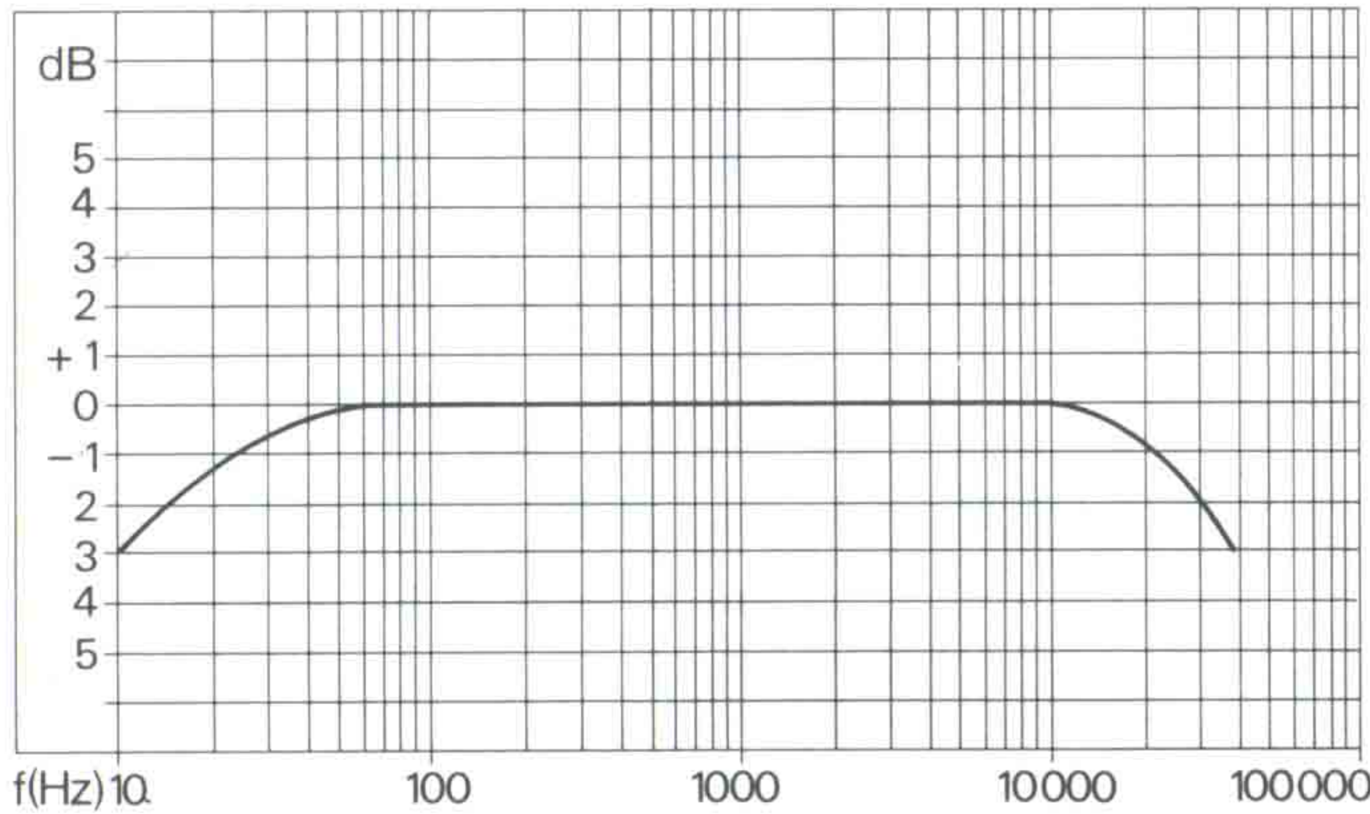
Fig. 3 Leistungsbandbreite nach DIN 45 500 10 Hz - 35 000 Hz
