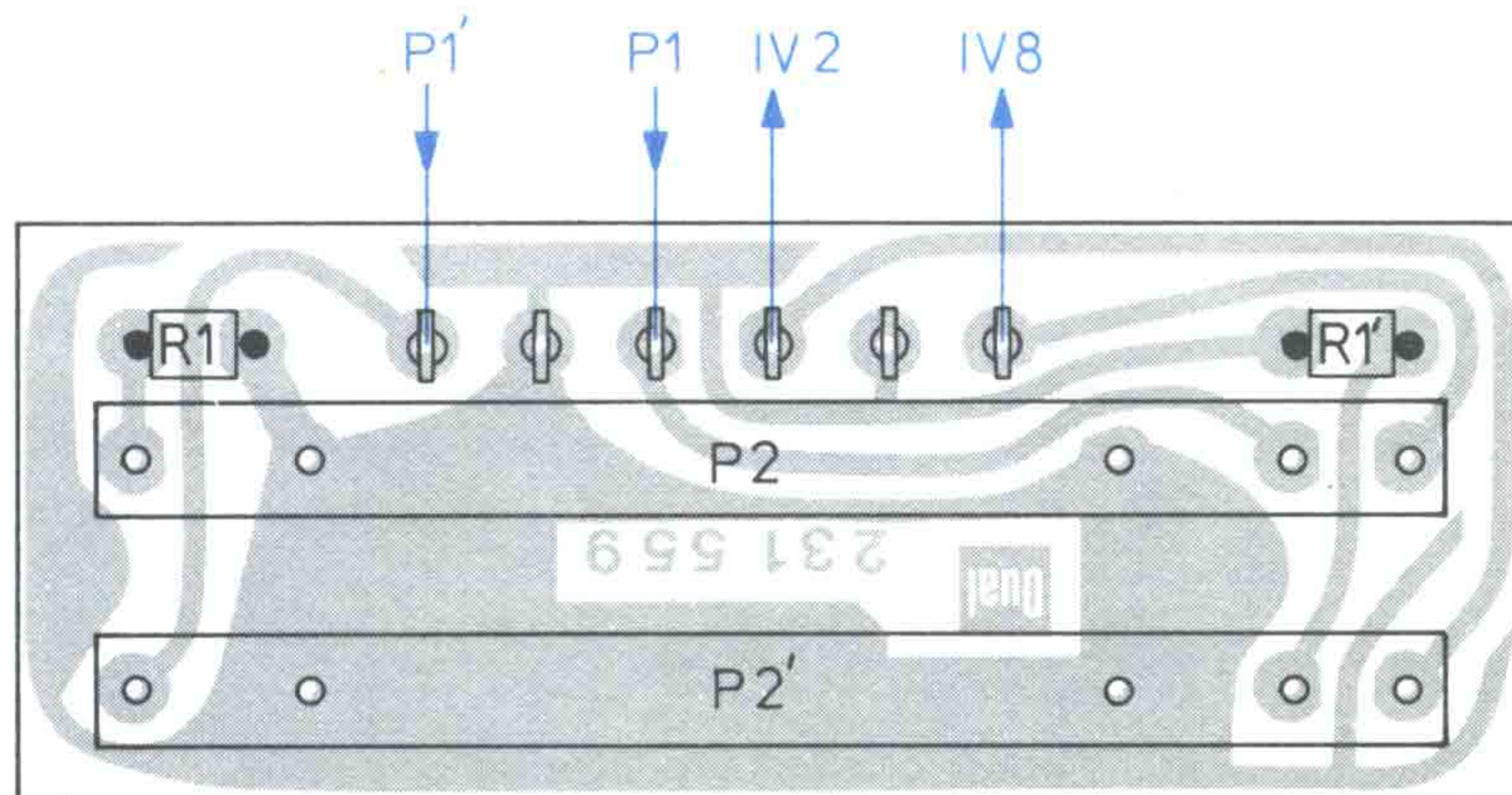
Fig. 9 Balancereglerplatte 233 989 (Leiterseite)
