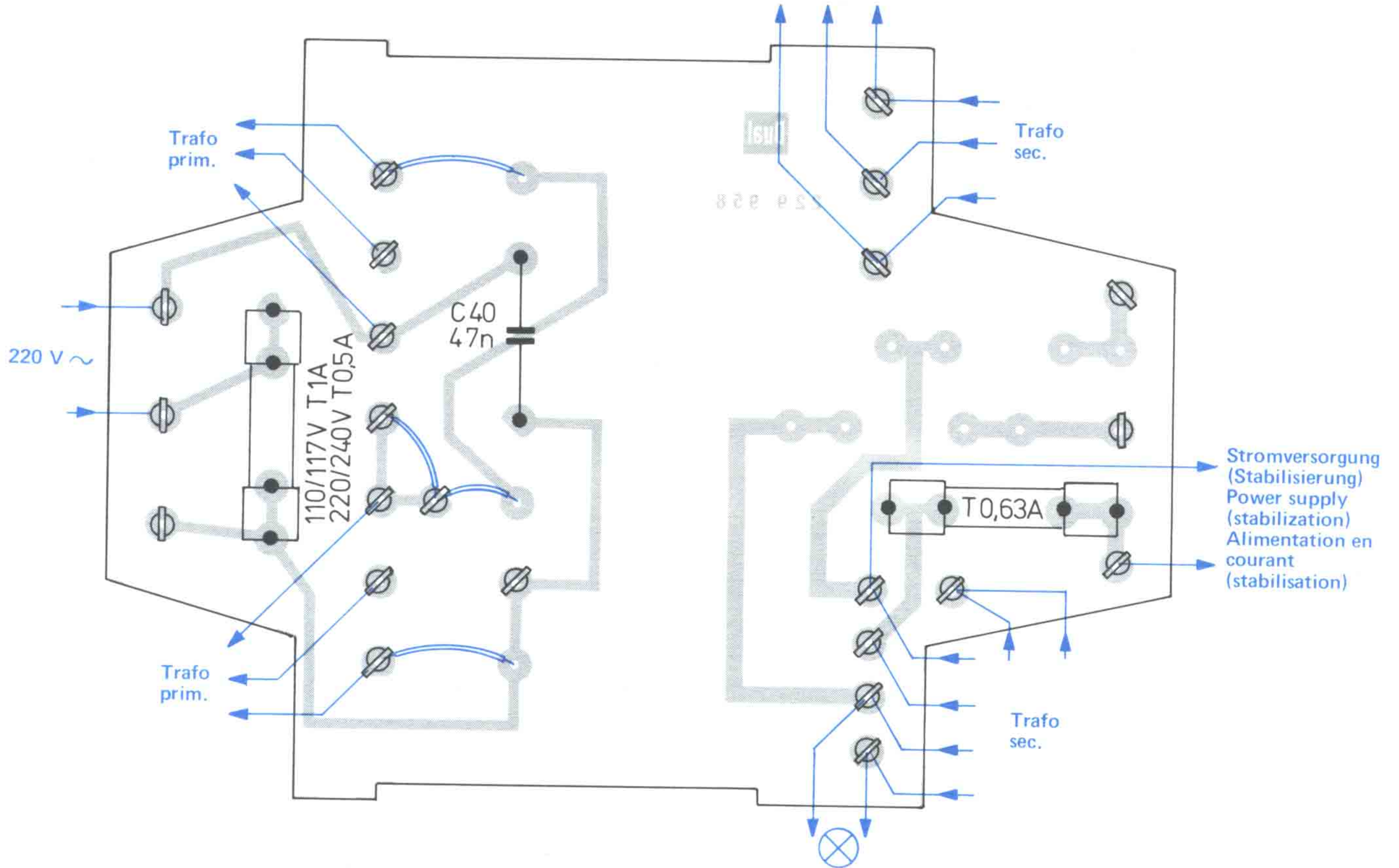
Fig. 11 Anschlußplatte 229 954 (Bestückungsseite) Endverstärker Power amplifier Amplificateur final
