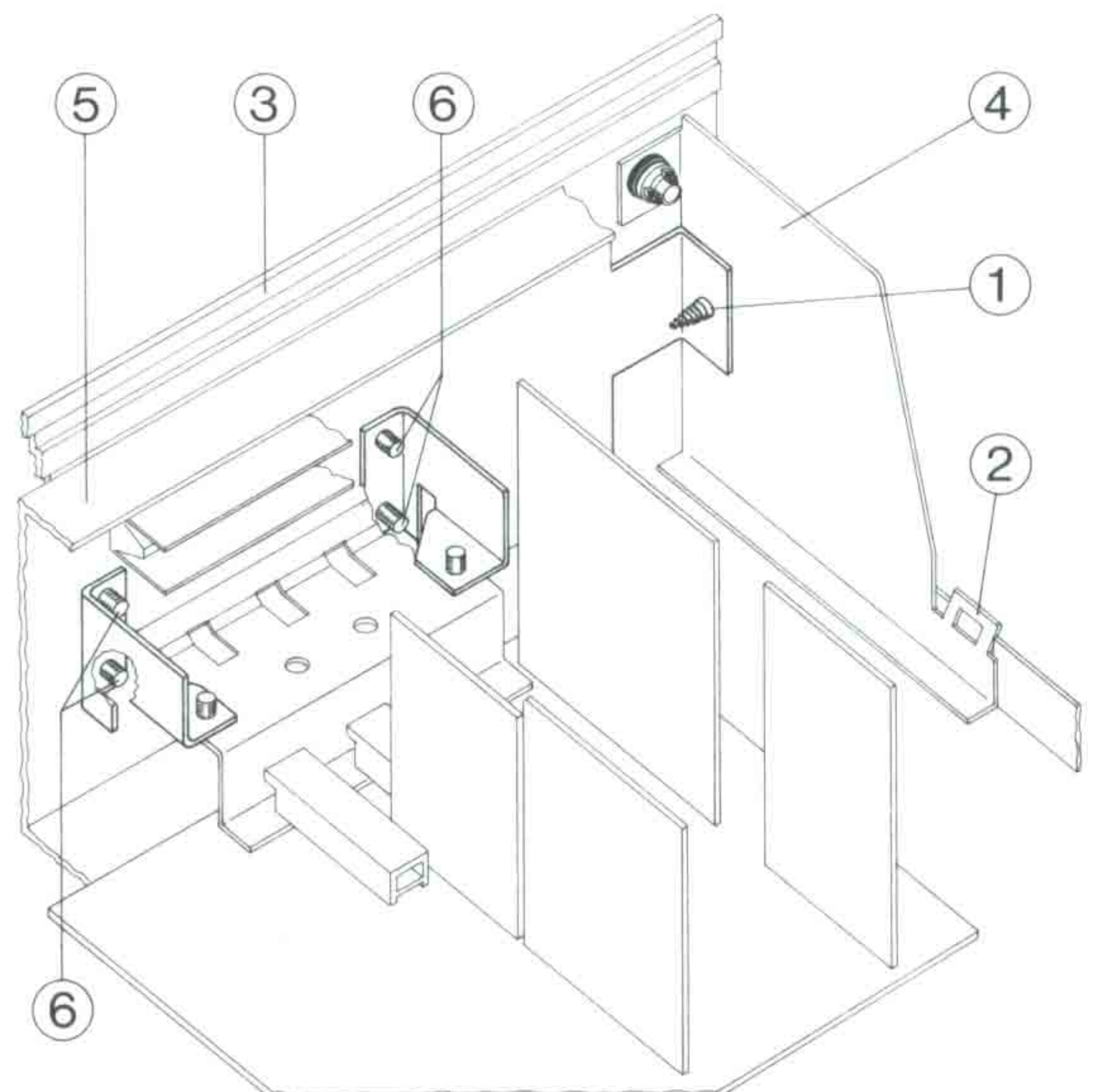
Fig. 26 Ausbau des Steuerverstärkers
