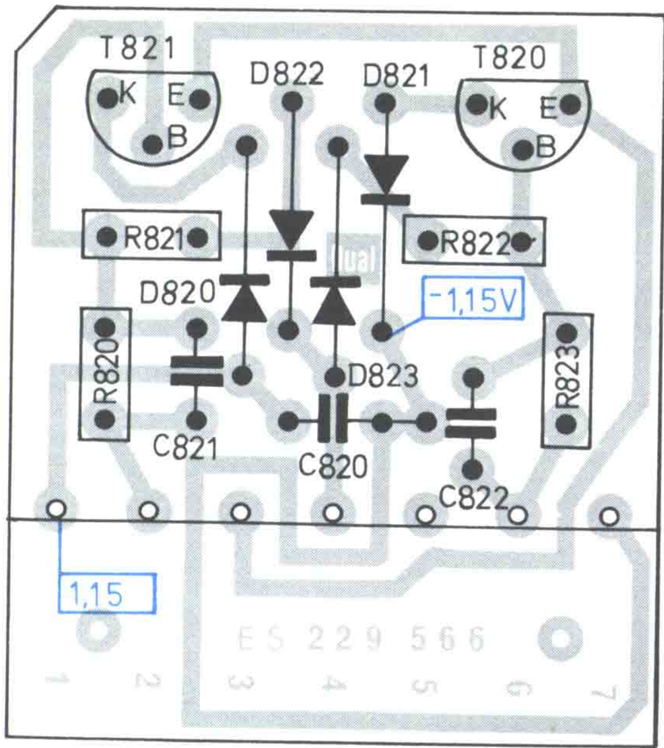
Fig. 23 Elektronische Sicherung VI 232 451 (Leiterseite)
