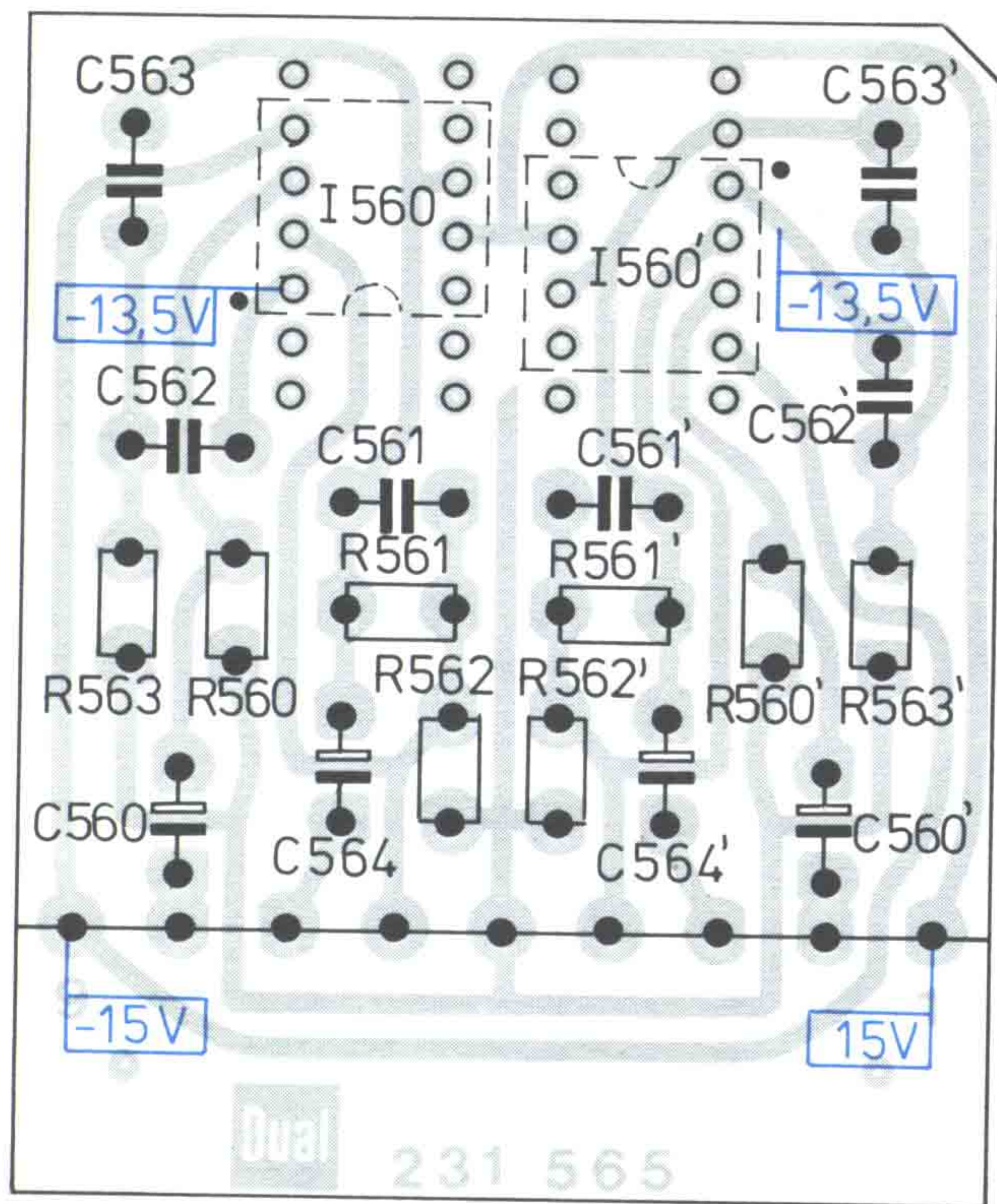
Fig. 19 Zwischenverstärker IV 233 991 (Leiterseite)
