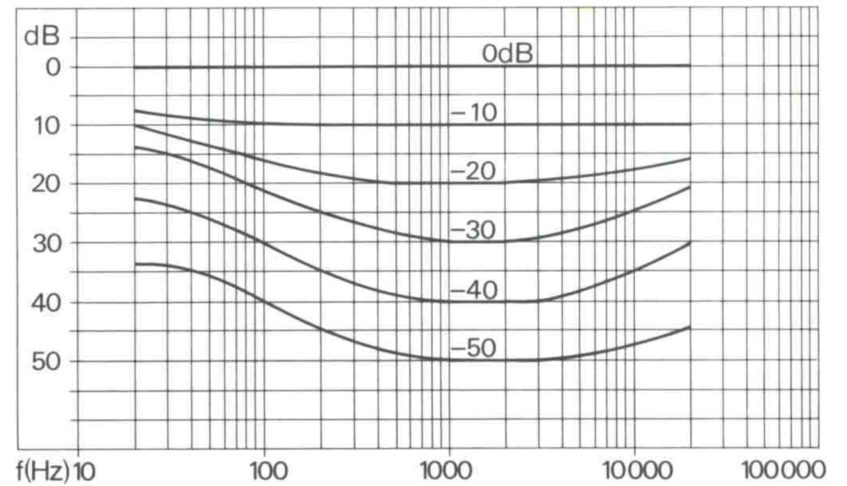
Fig. 6 Wirkungsweise der physiologischen Lautstärkeregelung 0 dB = Lautstärkeregler offen
