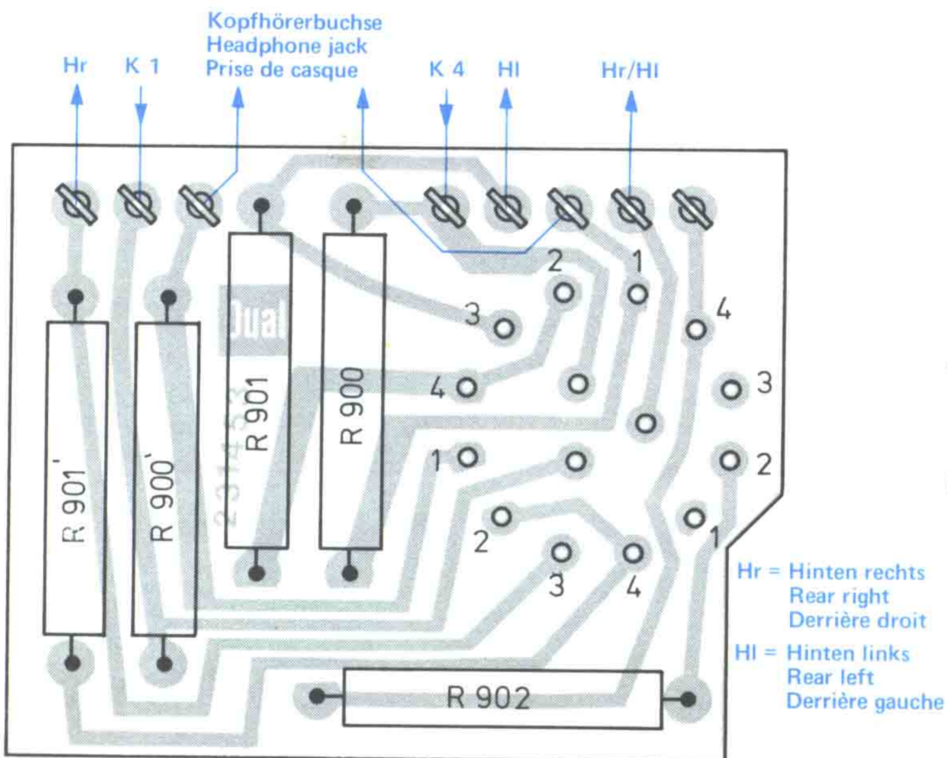
Fig. 25 Modeschalter 233 975 (Leiterseite)
