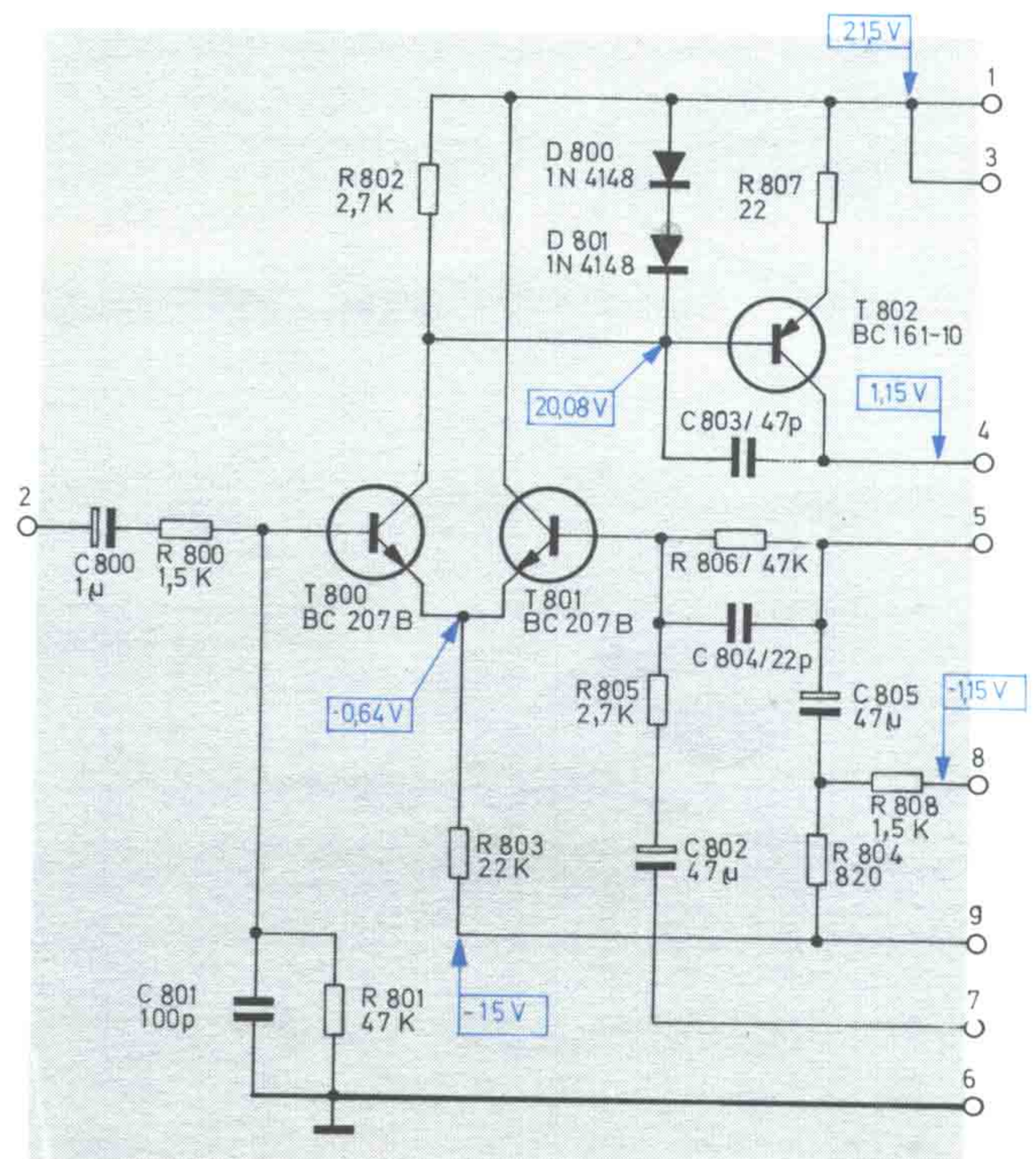
Fig. 22 Universalstreiber V Schaltbild
