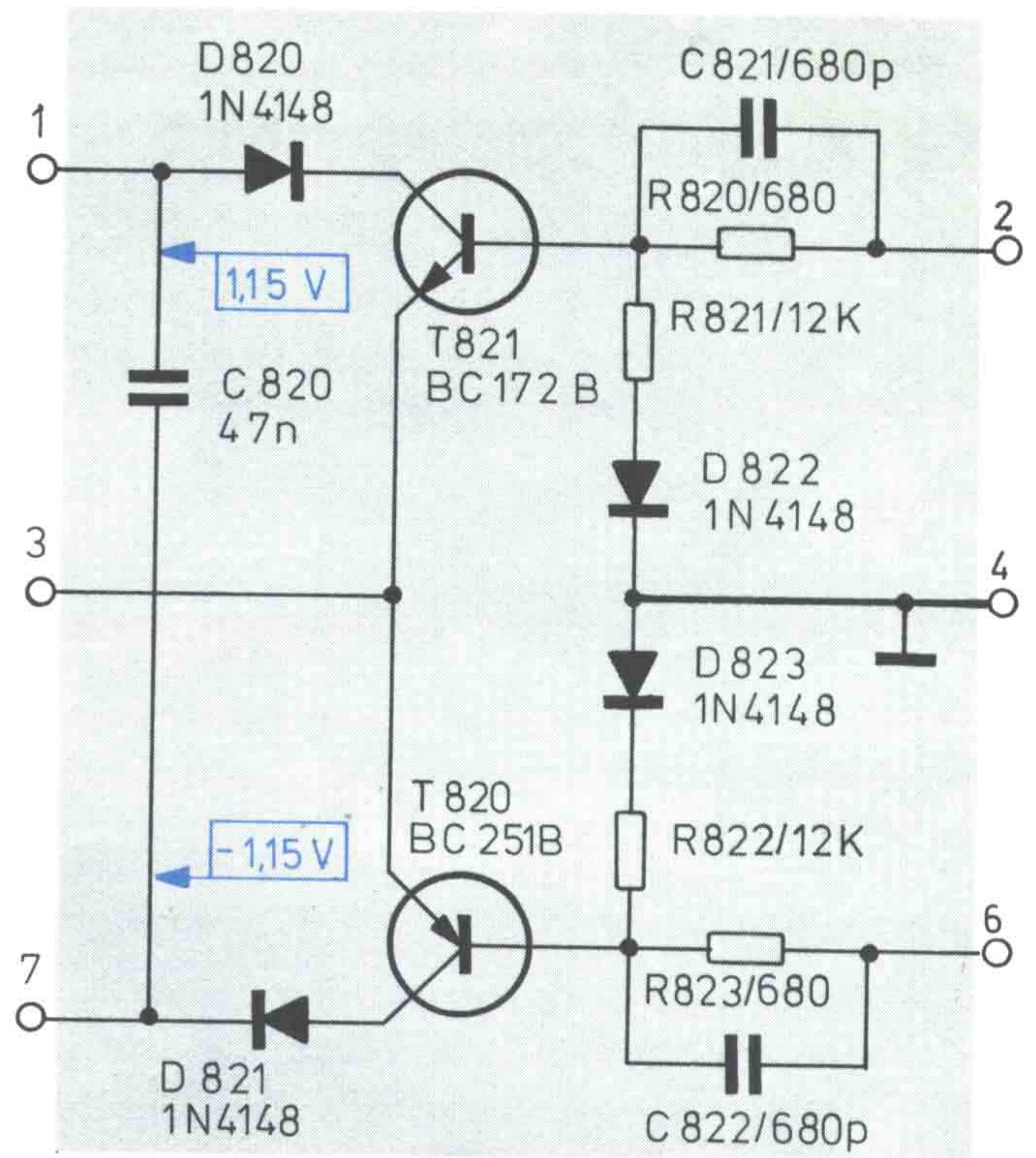
Fig. 24 Elektronische Sicherung VI Schaltbild
