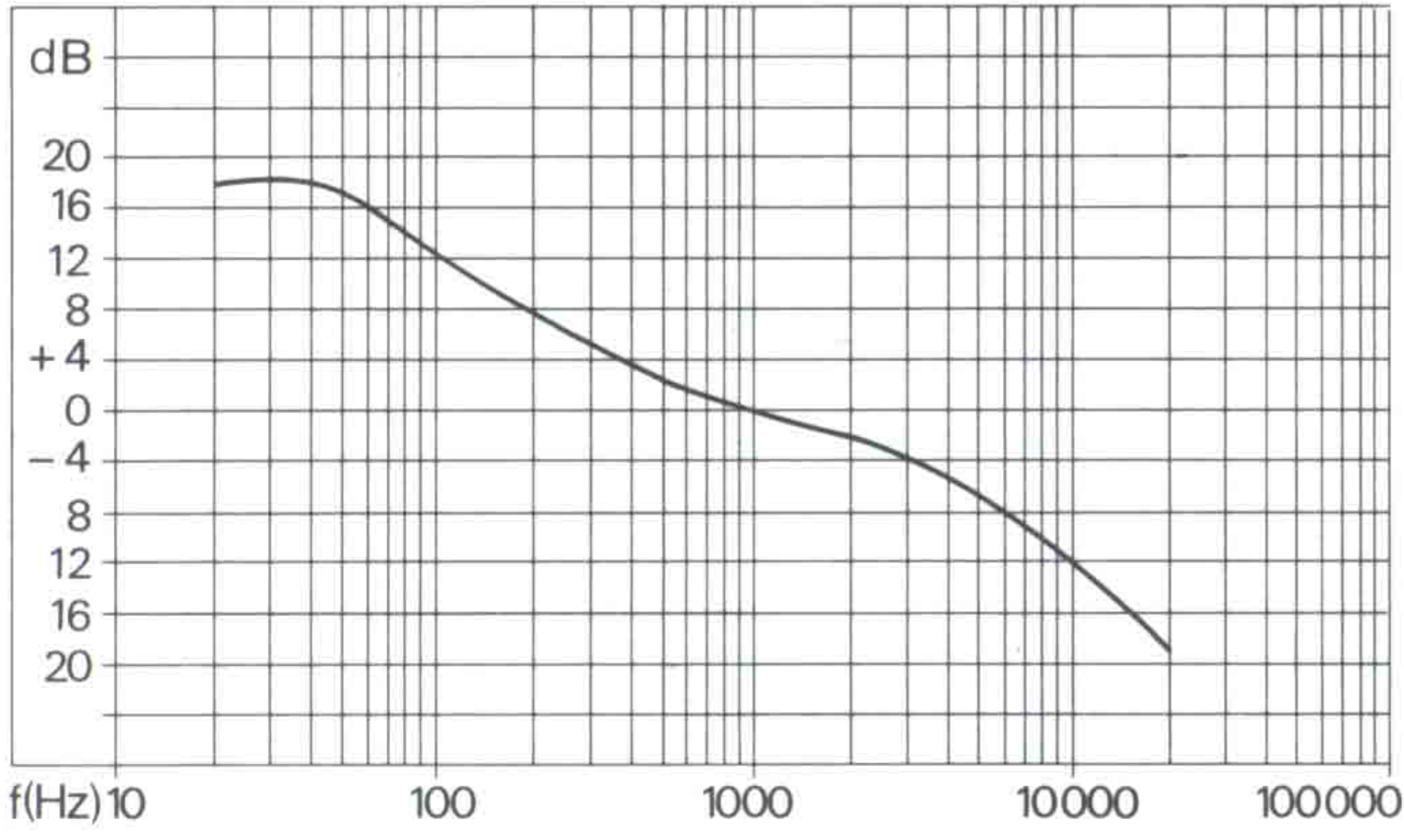
Fig. 1 Frequenzgang des Vorverstärkers Magneteingang
