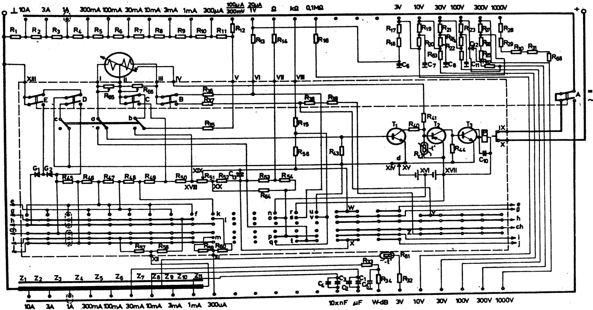
Obr. 8 Schéma vnitřního zapojení DU 20
