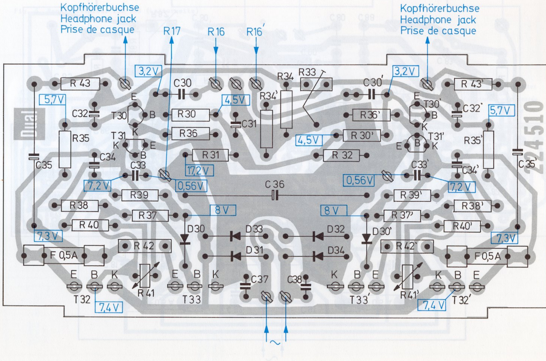
Fig. 3 Endverstärker 225 473 (Leitersseite)
