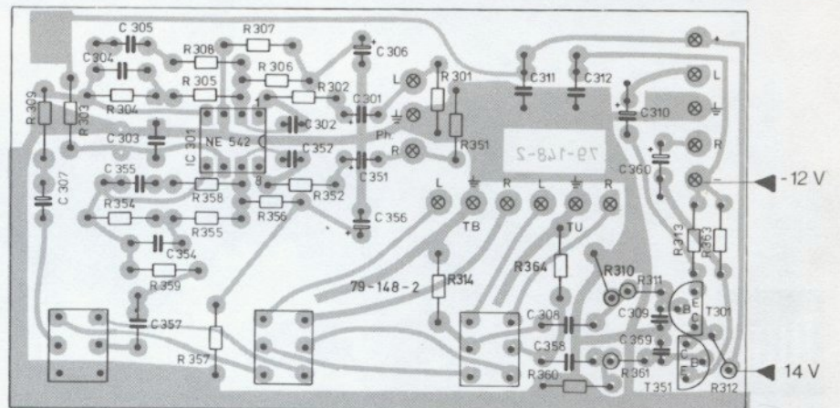
265 684 Phonovorverstärker Bestückungsseite
