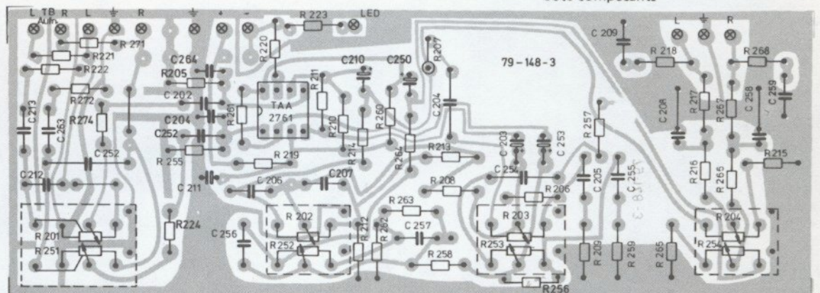
265 685 Klangreglerplatte Bestückungsseite Tone control board equipment side Plaque de régulateur de tonalité côté composants
