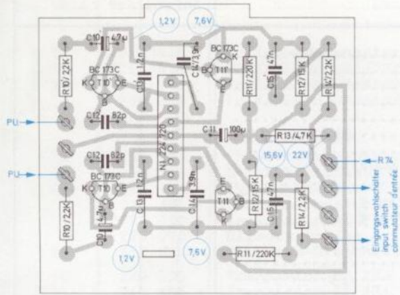
Fig. 2 Ätzsaltplatte des Vorverstärkers 227 585 (Leiterseite)
